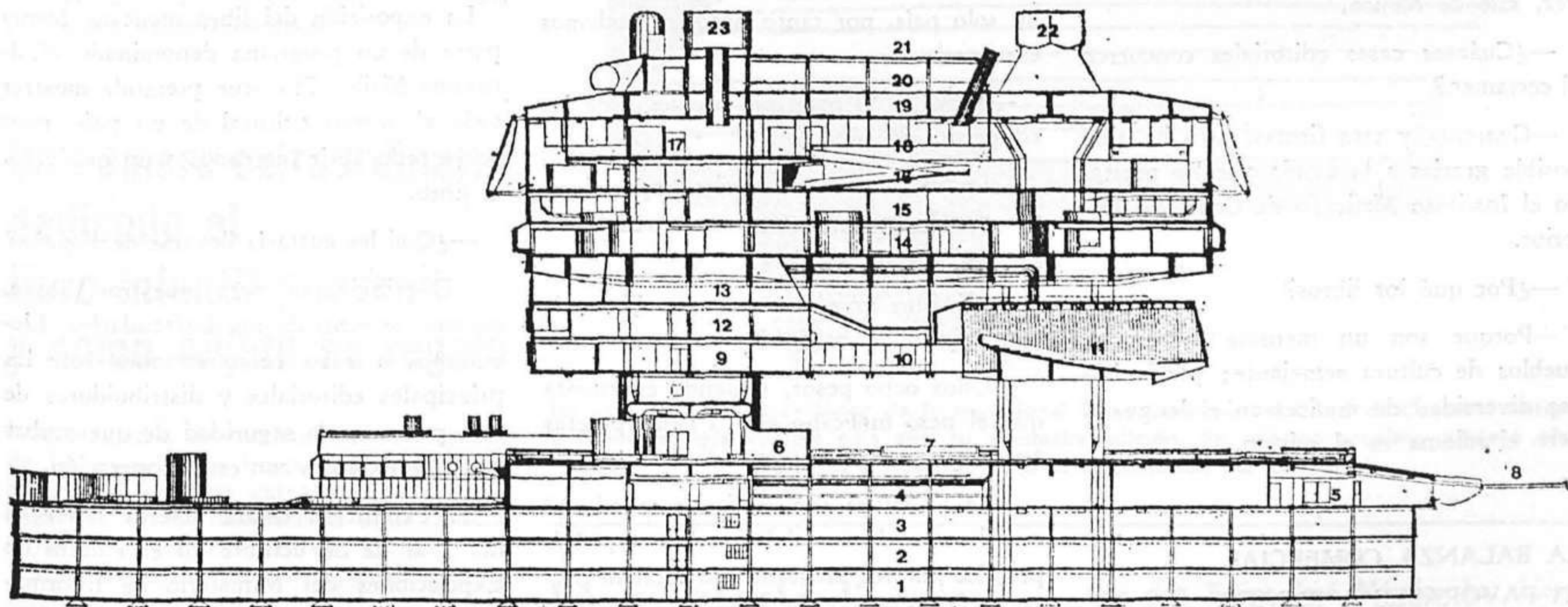
1. Tercer subsuelo, depósito de libros.—2. Segundo subsuelo, depósito de libros.—3. Primer subsuelo, depósito hemeroteca.—4. Hemeroteca.—5. Sala de publicaciones antiguas.—6. Hall planta baja.—7. Terraza cubierta.—8. Explanada.—9. Dirección.—10. Exposiciones.—11. Auditorio.—12. Administración.—13. Sala de máquinas.—14. Salas especiales.—15. Depósito de salas especiales.—16. Salón de lectura.—17. Hall de acceso al público.—18. Referencia.—19. Sala superior de máquinas.—20. Pasarela.—21. Azotea.—22. Sala de máquinas de los ascensores.—23. Tanque de agua.
