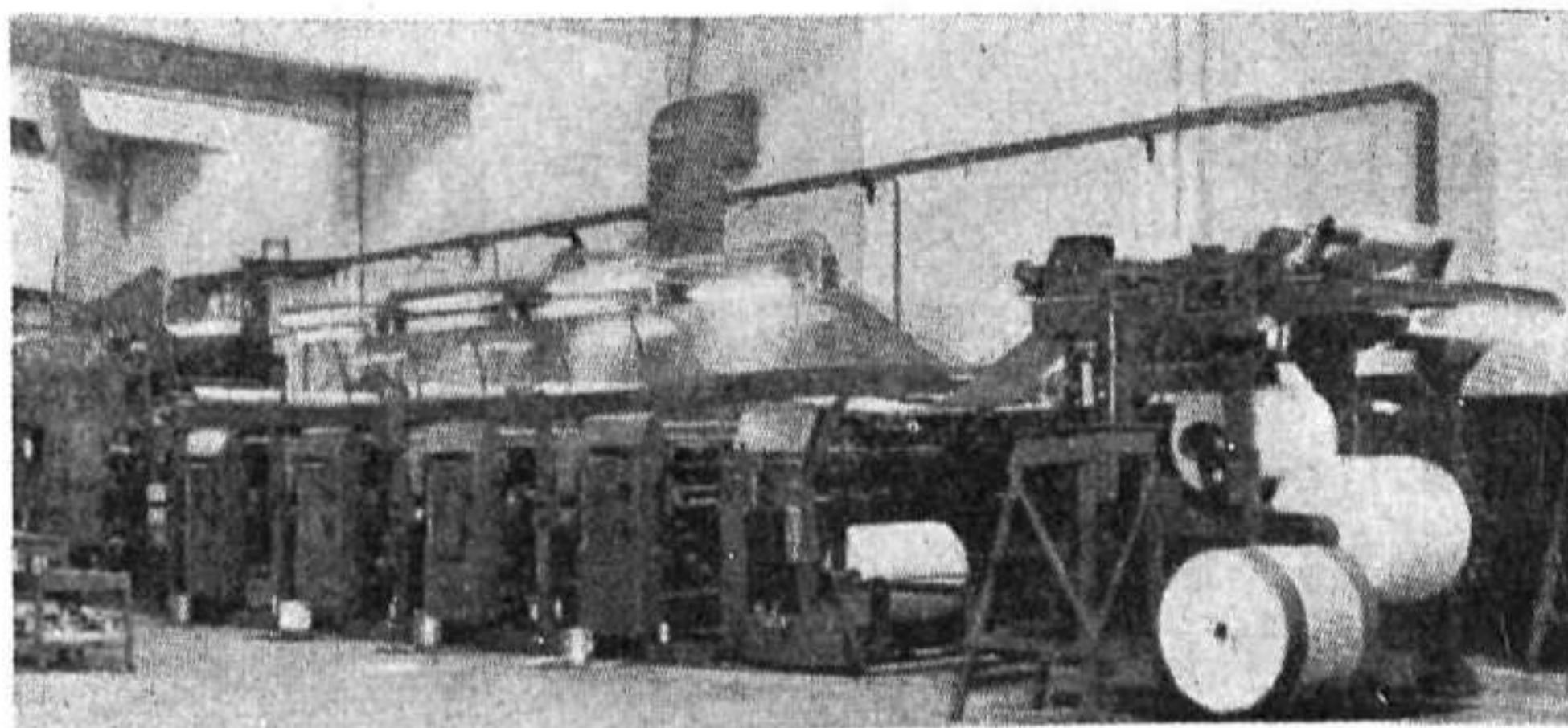
La moderna rotativa HARRIS-COTTRELL que imprime a la vez ocho tintas (cuatro por cada lado) con una velocidad promedio de 16,000 pliegos impresos y doblados por hora
