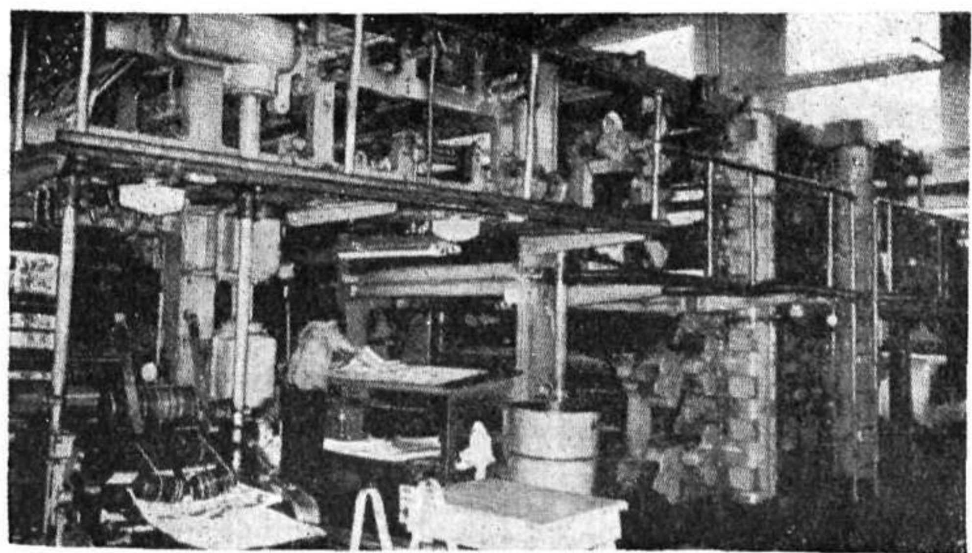
Rotativa HOE de ocho colores (cuatro por ambas caras) que imprime y dobla dos revistas distintas a la vez, de 32 páginas cada una, produciendo 40,000 revistas por hora
