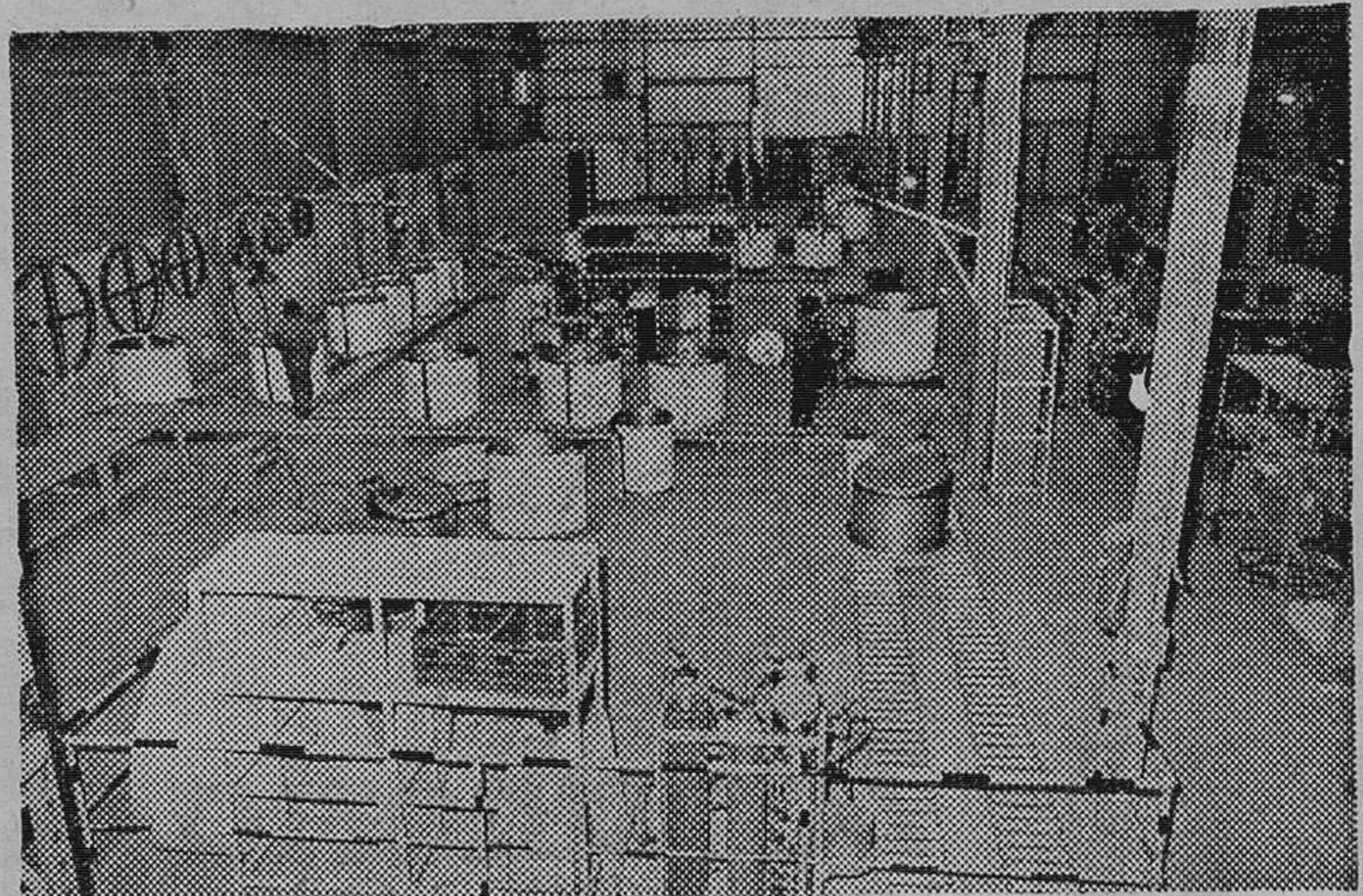
Esta es la cadena de fabricación de los tanques; el proceso comienza en la parte inferior de la fotografía y el producto queda acabado al fondo, donde existe una unidad de prueba. — (Foto FEDE)
