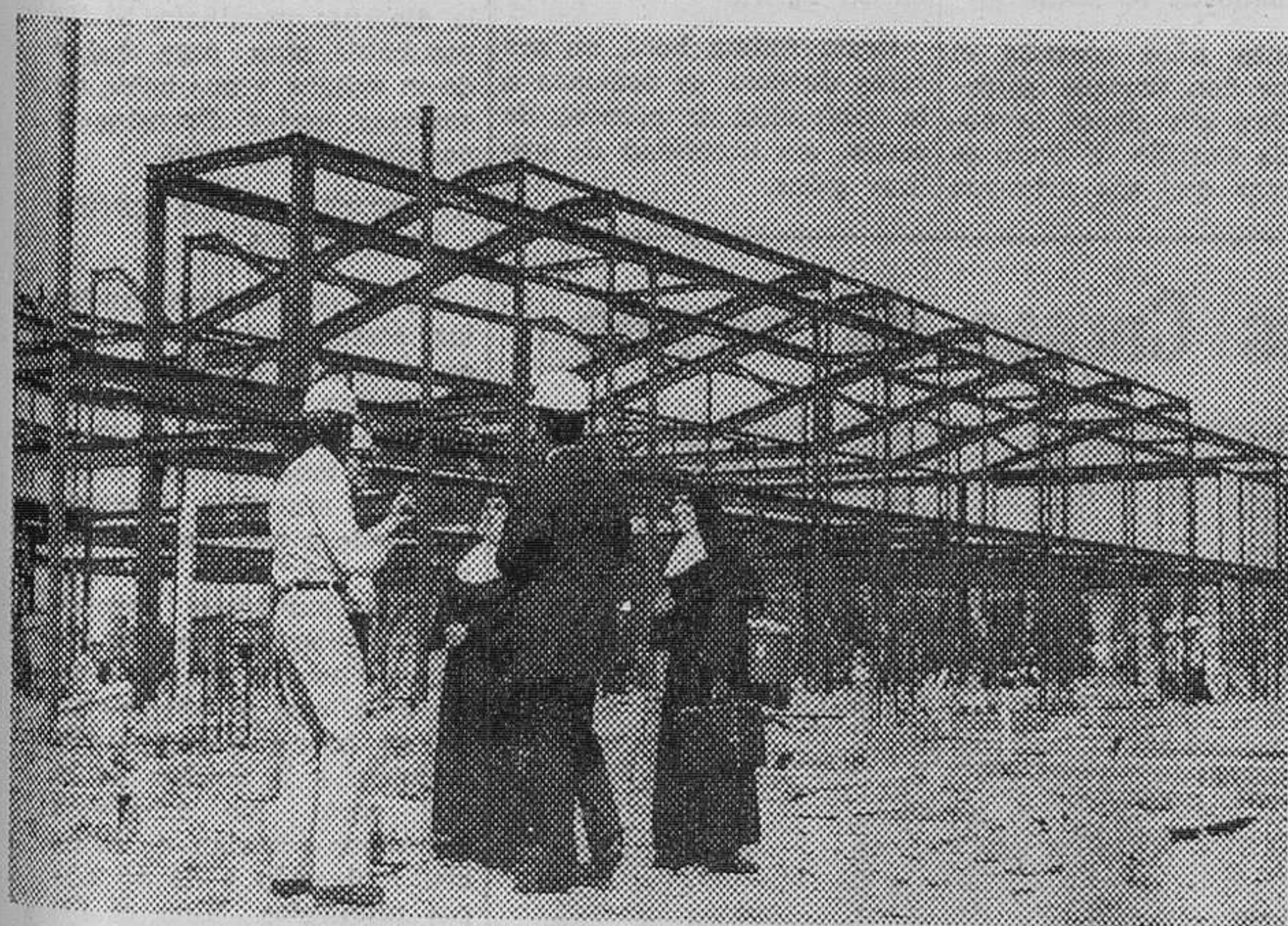
Religiosas, técnicos de la obra e informador conversan animadamente al pie de la obra de la Residencia-Hogar que hoy comienza a adquirir formas en el simétrico juego de sus estructuras metálicas que son como el esqueleto de un armonioso cuerpo arquitectónico destinado a hacer feliz la ancianidad de los desamparados. (Foto FEDE)
