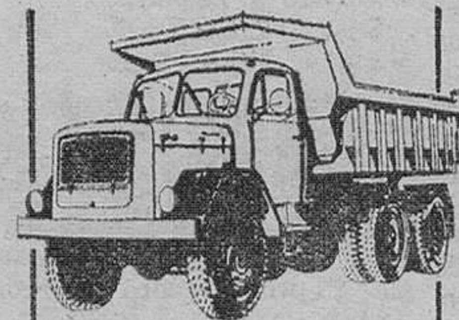
DUMPER Tres ejes tracción total 230 D 26 AK 6 X 6 DE 250 C.V.
