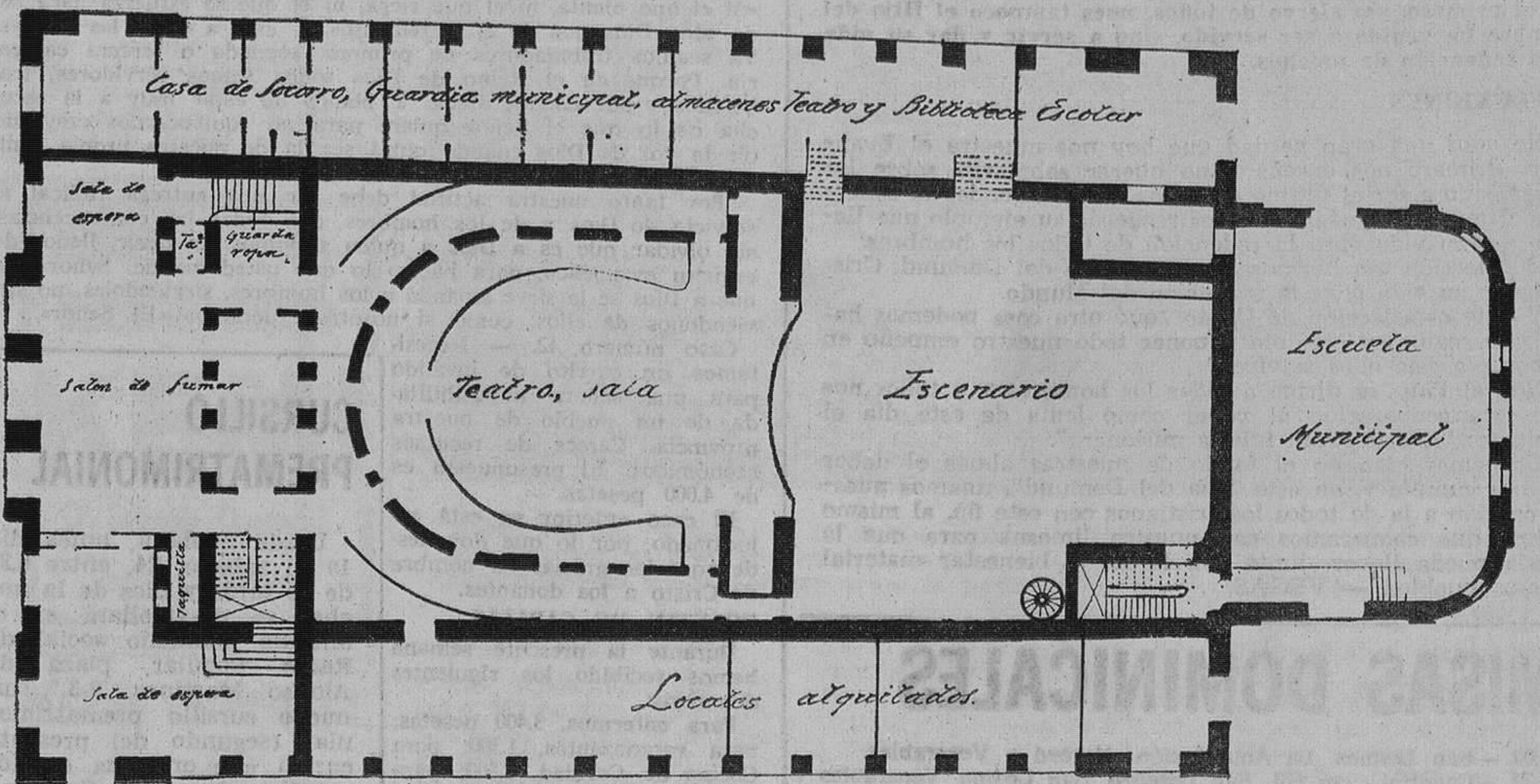
Planta del Teatro Principal y distribución de sus locales, por los años veinte
