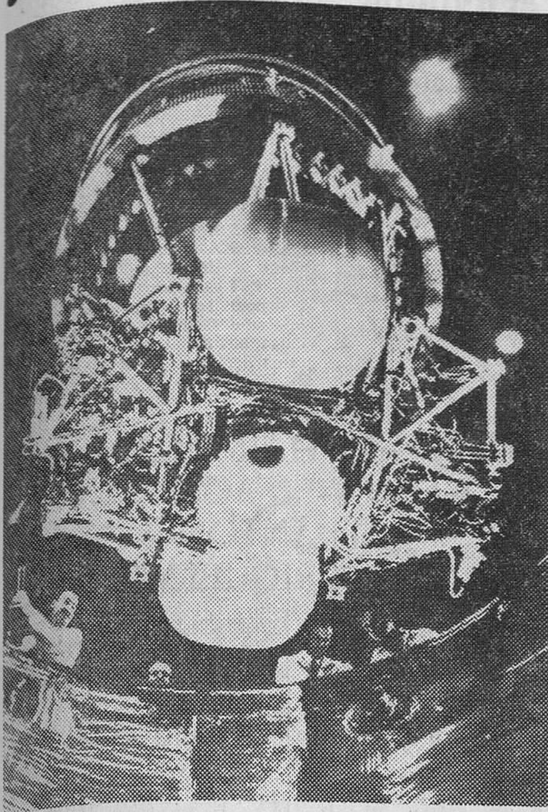
Siete países, docenas de organismos oficiales y casi un centenar de empresas trabajan en la construcción del proyectil portador "Europa 1" de la ELD... (Foto Fiel)
