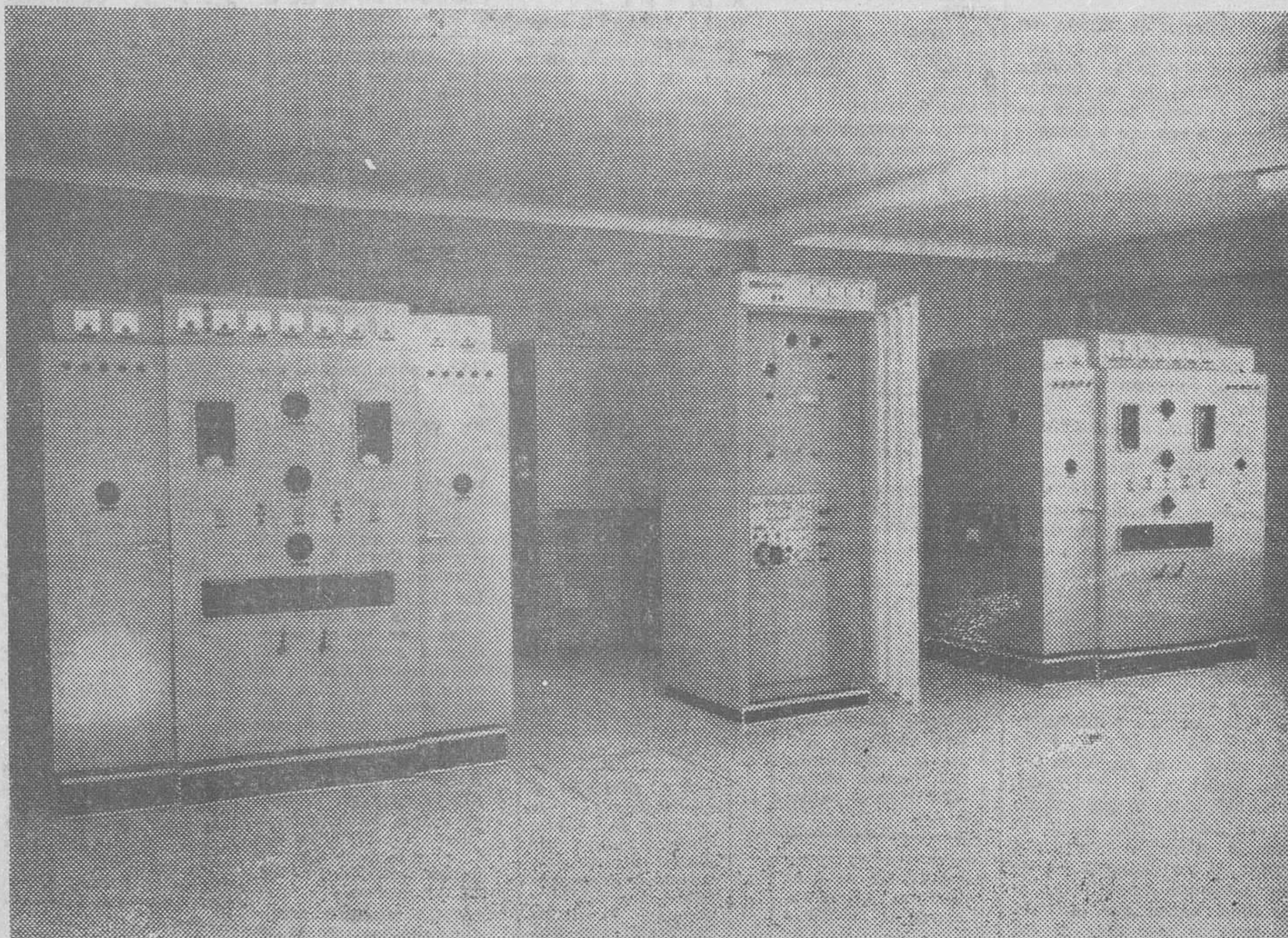
HE AQUÍ UN CONJUNTO TÉCNICO DE CARA AL FUTURO. TODOS LOS SERVICIOS SON DOBLES. DOS LINEAS DE ALTA TENSION, DOS EMISORAS, LISTAS PARA UNA SUSTITUCION INMEDIATA —10 SEGUNDOS— Y MULTIPLE CONEXION TELEFONICA, CONSTITUYEN PLENA GARANTIA DE UNA EMISION PERFECTA EN CALIDAD Y SIN INTERRUCCION.
