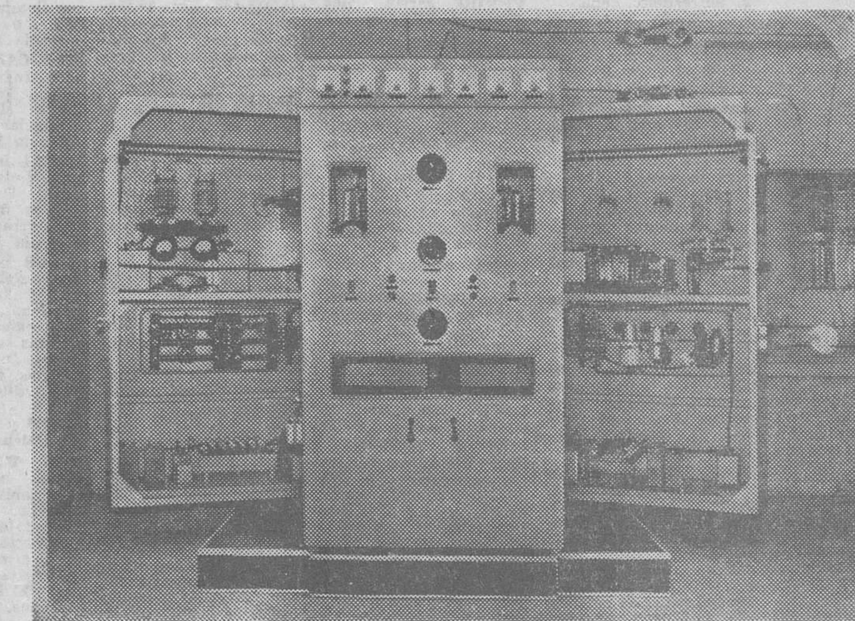
UNA DE LAS EMISORAS DE ONDA MEDIA (2,5 K.W.)
