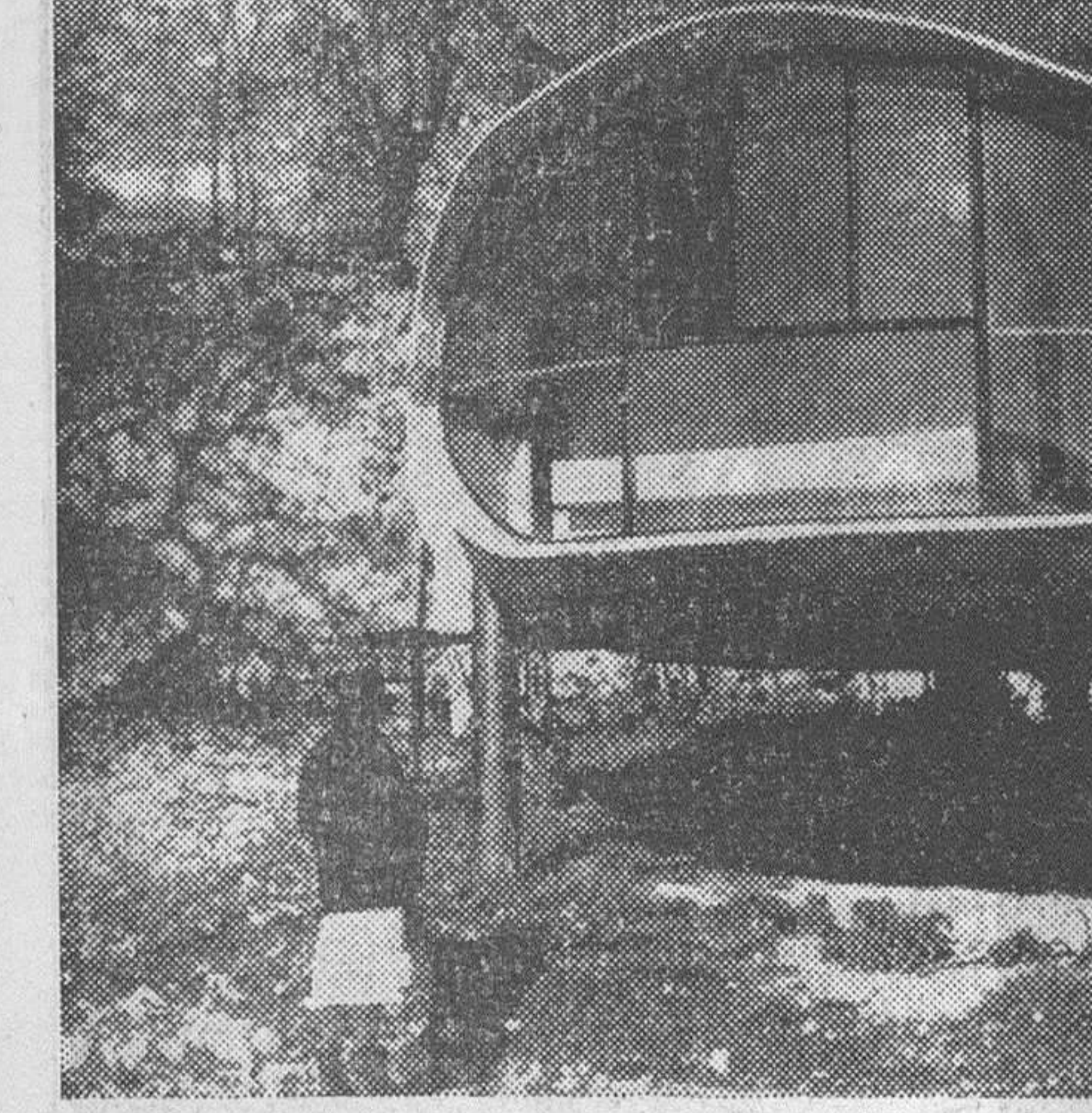
Una campesina contempla asombrada, cerca de Ginebra, la vivienda de plástico, en forma de huevo, obra del arquitecto suizo Pascual Hauserman. Consta de dormitorio, cocina y baño, pesa sólo de 600 a 800 kilos y los tres soportes sobre los que se sienta hacen que se acomode a todos los terrenos. (Foto Fiel)
