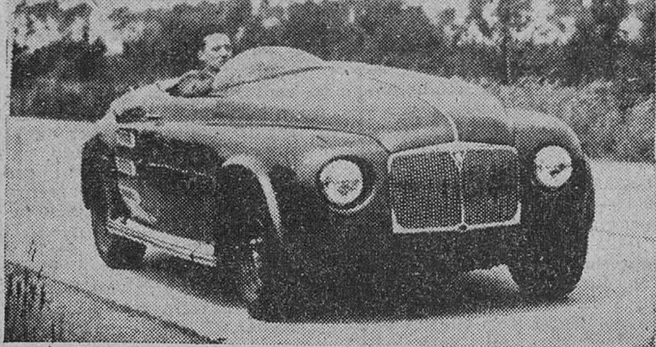
El "Rover" de turbina de gas. Se aprecia la entrada de aire en la parte posterior del vehículo.
