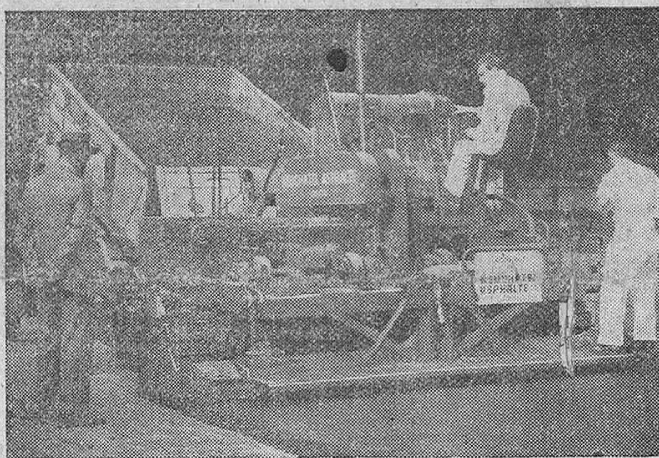
Esta máquina que se utilizó para construir aeródromo, durante la guerra, se emplea ahora en Inglaterra para el trazado de nuevas carreteras. Esparea el asfalto de manera uniforme y lo iguala cualquiera que sea la desigualdad del suelo. A medida que avanza va dejando la calzada ya terminada.—(Foto Cifra)
