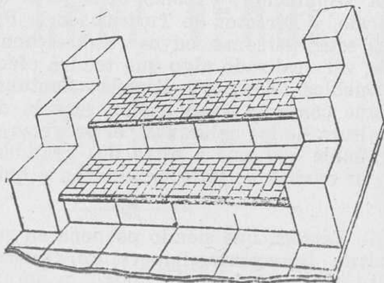
Escalera con pasos antirresbalable "CRESPO"
