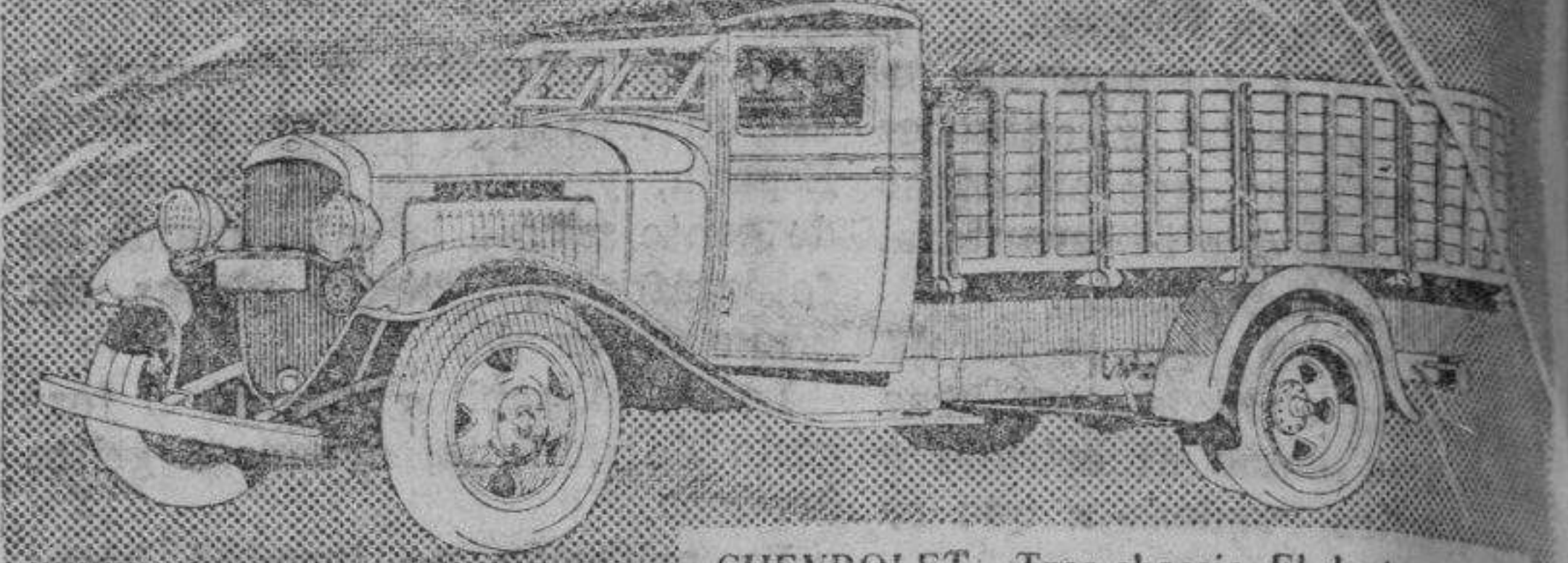
CHEVROLET.—Tres chasis. El de 4 mts. entre ejes, 2 1/2 toneladas de carga útil, balastos múltiples, ruedas gemelas con neumáticos 32 x 6 reforzados. Ptas. 10.950
