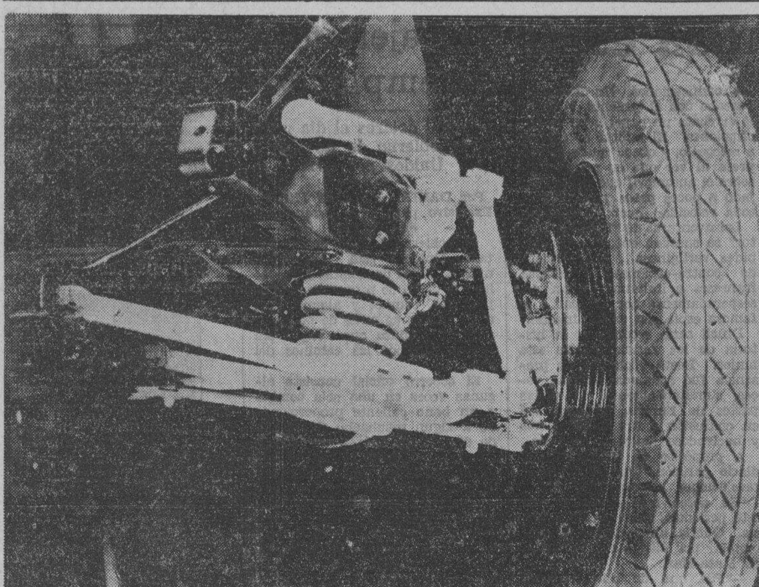
La comodidad que se encuentra en los automóviles Buick de 1934 se explica con estos muelles con acción de efecto de rodillas, que permite un movimiento independiente para cada una de las cuatro ruedas. Los muelles son de acero bien templado, y no solamente dan confort a los pasajeros sino que también protegen al coche de las tempranas roturas.
