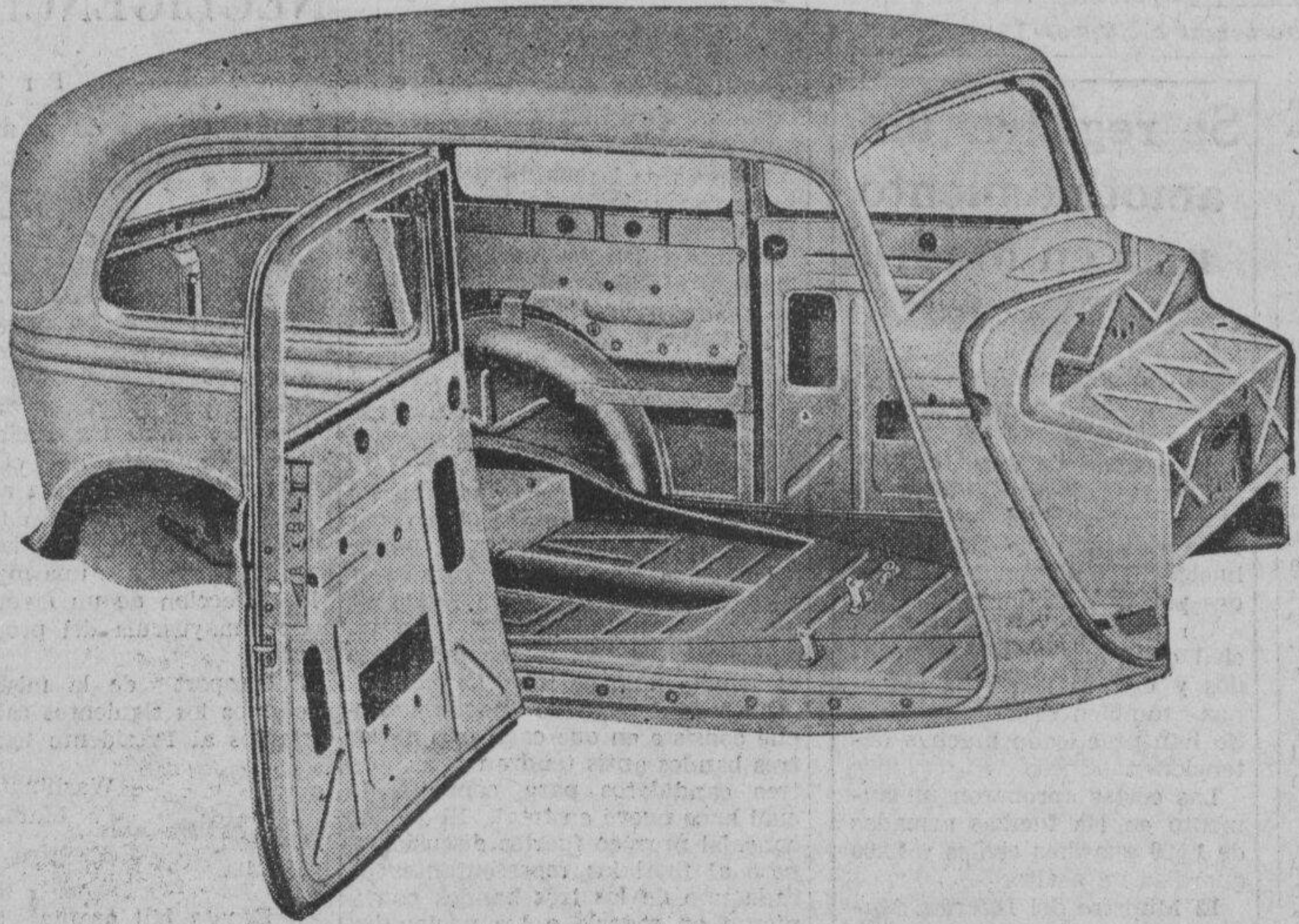
Esta es la forma de la armazón toda hecha de acero y con todas las partes unidas entre sí con soldadura eléctrica del Ford V-8 de 1934. Esta practica evita el empleo de la madera que en países tropicales como este se tiene que cambiar periódicamente y cuesta mucho dinero, además de hacer del coche mas duradero y mas resistente contra posibles accidentes.
