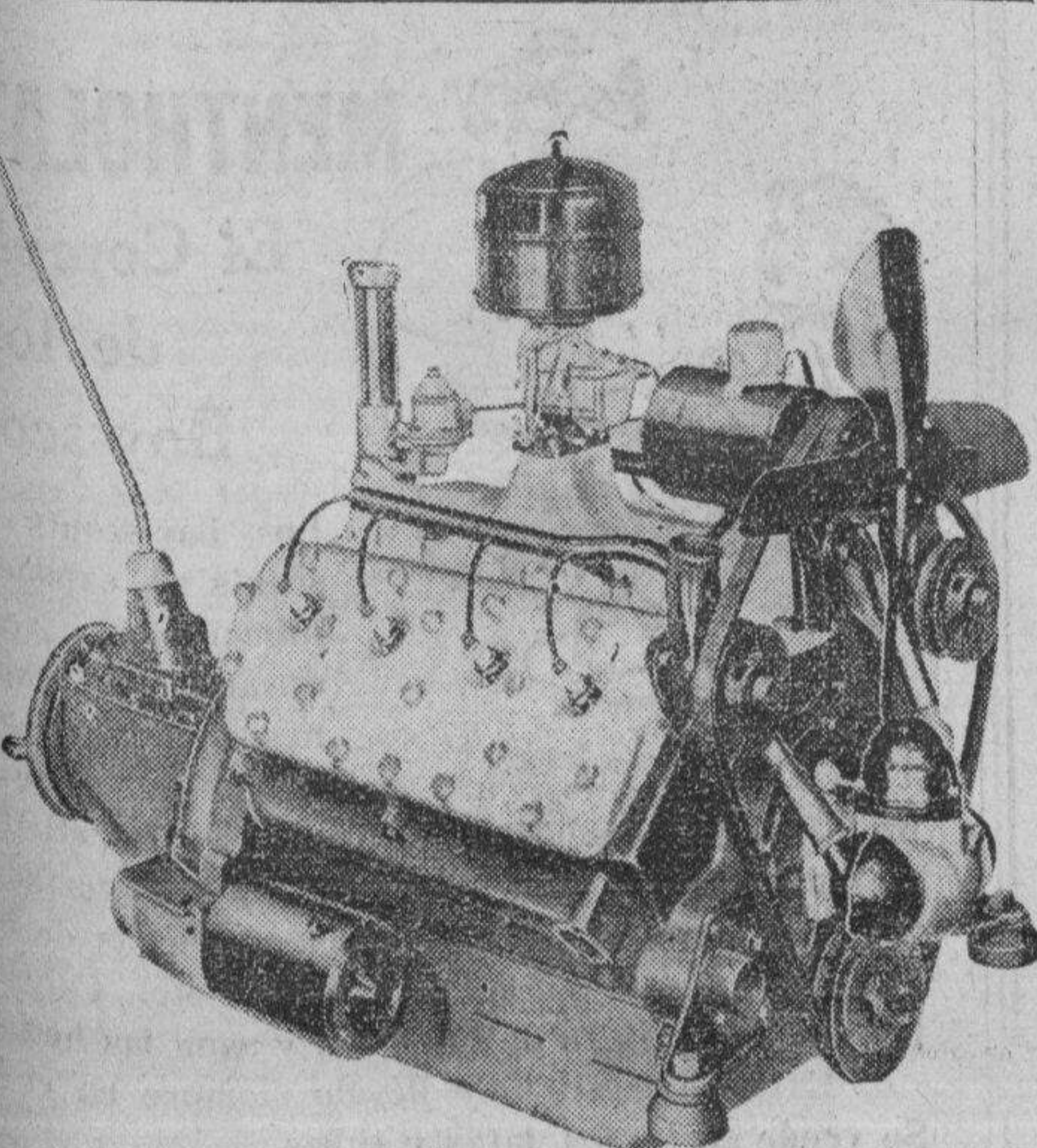
Este es el nuevo motor grandemente mejorado del Ford V-8 de 1934. En potencia, aceleración y suavidad, este motor no tiene igual.
