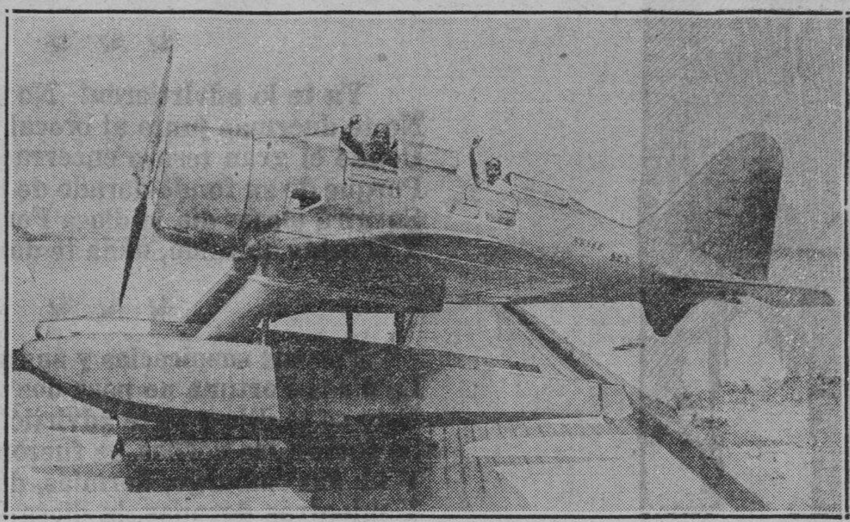
Este avión considerado como el mas veloz en todo Estados Unidos, ha sido diseñado por el Comandante Alexander P. Seversky, aviador ruso. Es destinado por su diseñador para usarlo en las carreras de aeroplanos para obtener el premio Bendiz de $100,000 de Nueva York a Los Angeles. El avión que es hidroplano y aeroplano a la vez, aparece con el Comandante Seversky manejándolo.
