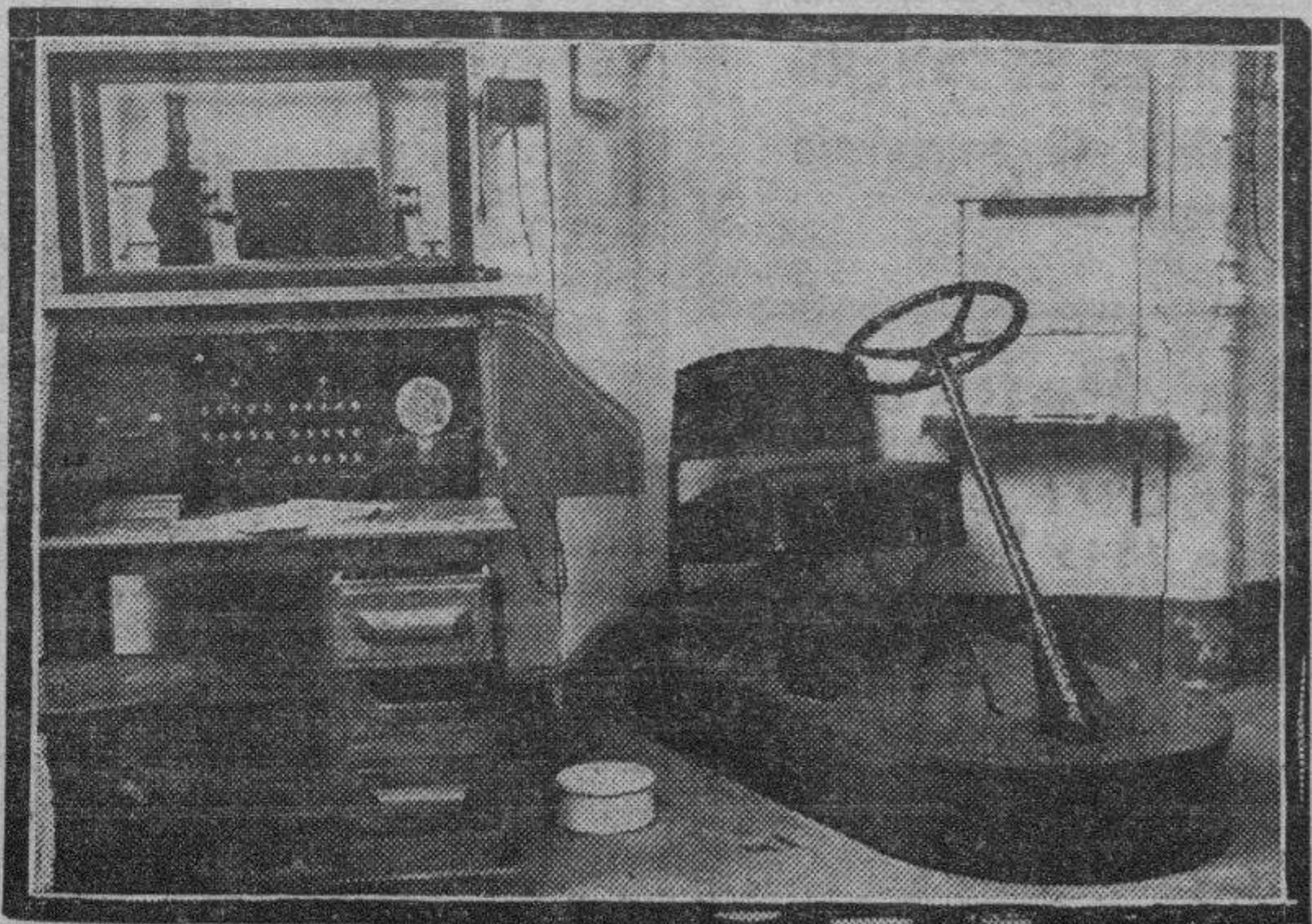
Aparato registrador de las perfectas maniobras y reacciones del chófer ante el peligro
