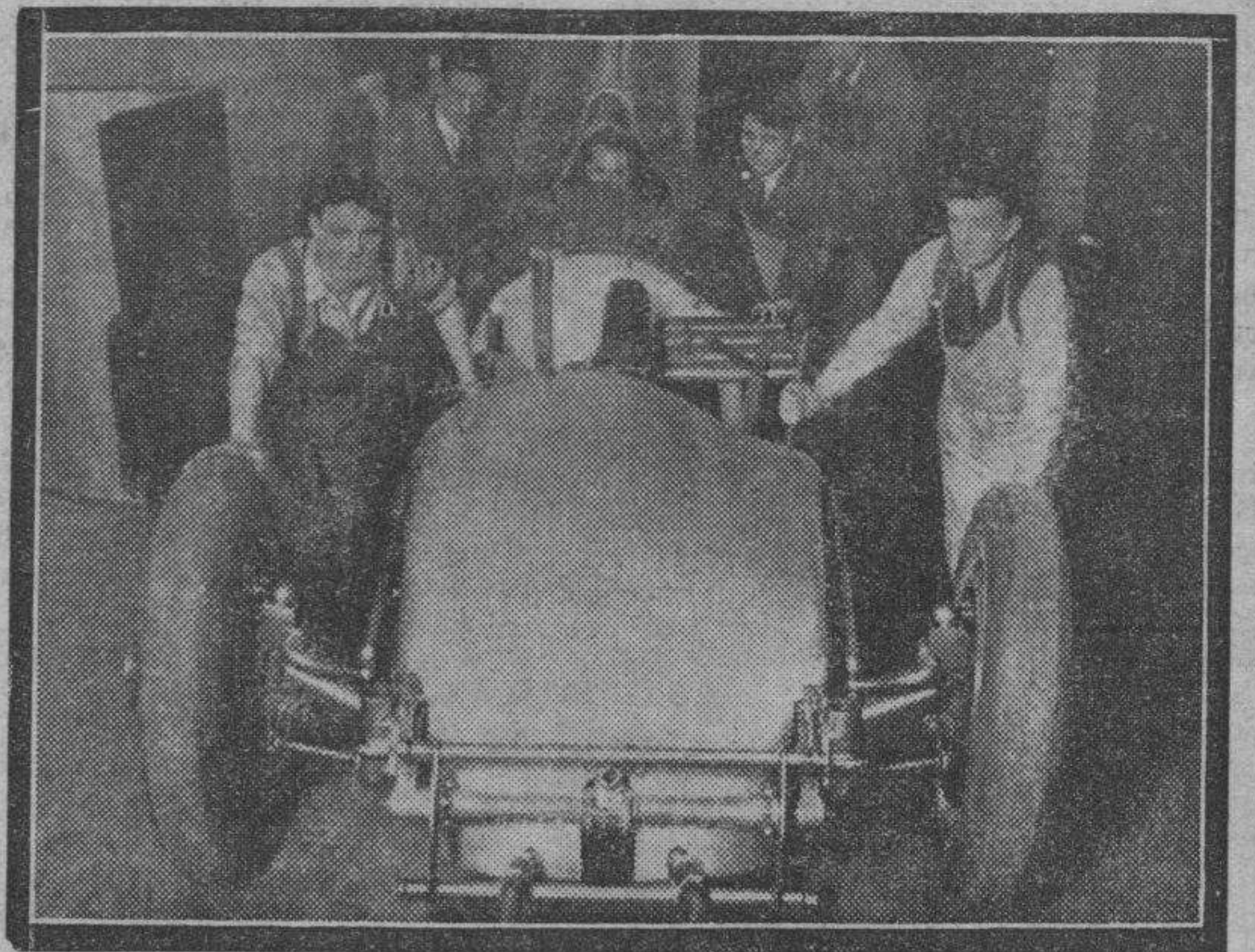
El nuevo "Pájaro Azul", en el que el capitán Campbell intentará batir el "record" mundial de velocidad de 231 millas por hora, que ostentó el difunto Seagrave.
