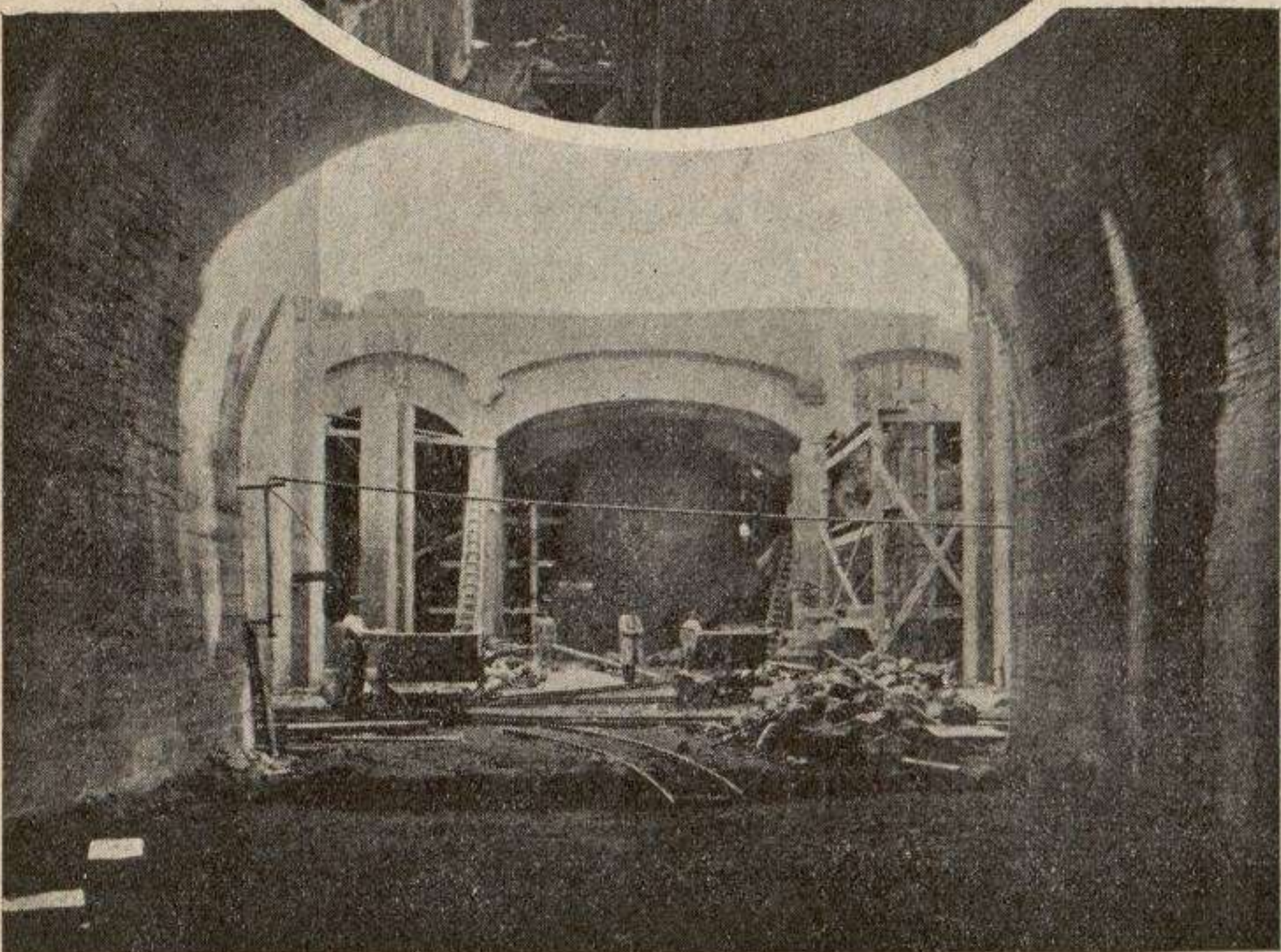
(Foto. superior) Muro de contención provisional para el cambio de rasante del f. c. en la estación de San Gervasio.
