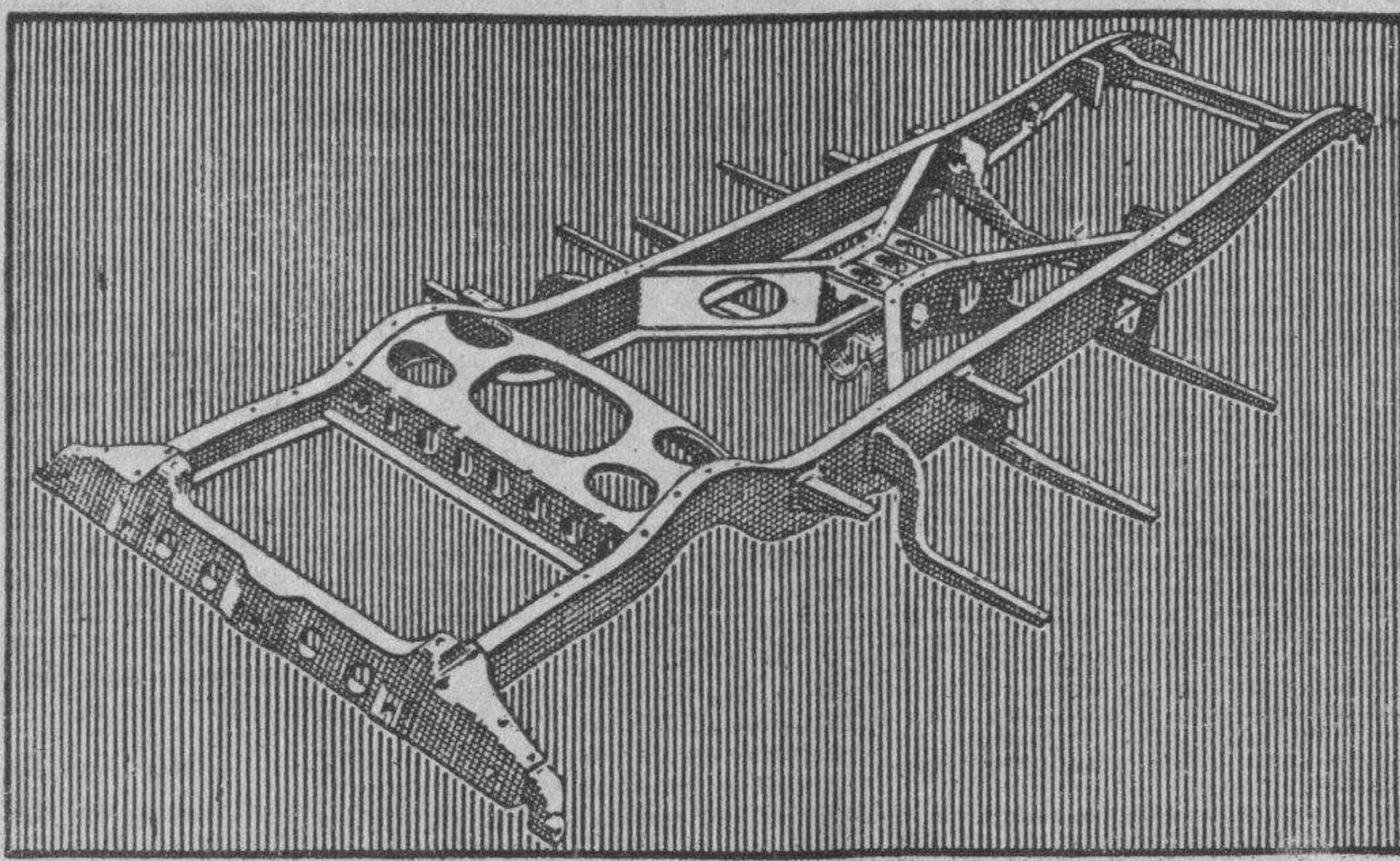
Bastidor del nuevo Essex, reforzado en X, igual sistema que el empleado en los carros de alto precio.
