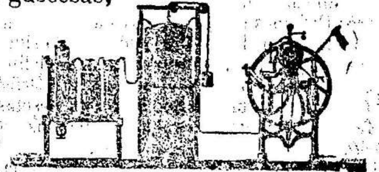
Aparatos para gaseosas. continuo, con embotelladoras puestas.
