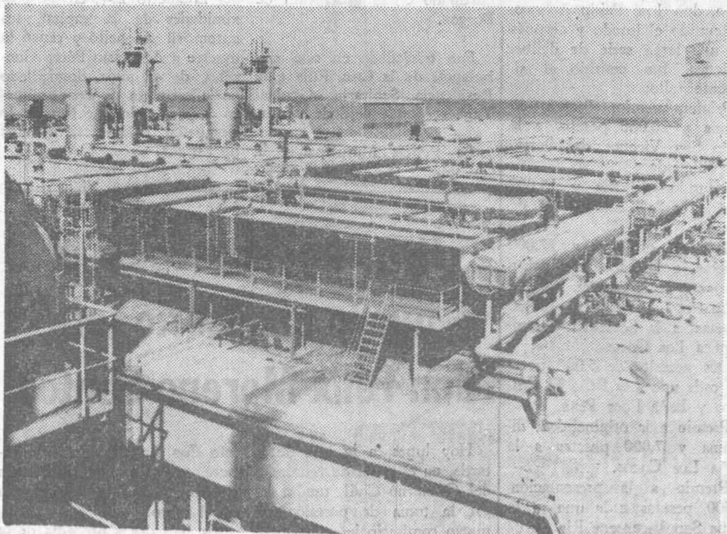
La central de agua potable ubicada en Zucitina (Libia) y construida por un consorcio industrial alemán, constituye el mayor complejo de desalinización de agua de mar construido hasta ahora. Aplicando el método de evaporación en diversas fases, la citada central alcanza una producción diaria de 10.000 metros cúbicos de destilado.
