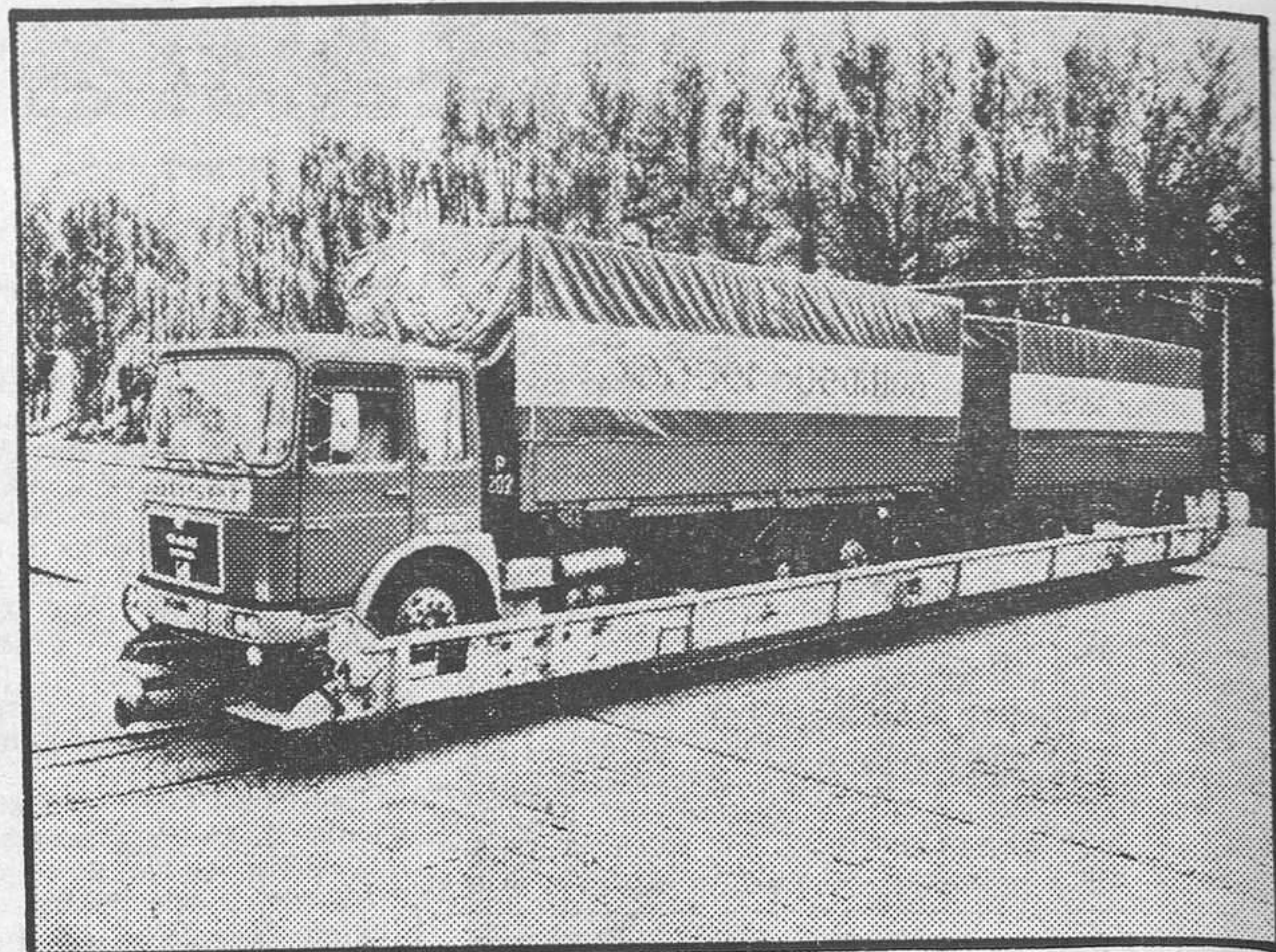
Francfort (DaD). — La fábrica alemana de vagones de ferrocarril «Talbot», de Aquisgrán, ha dado su nombre a este nuevo vagón de carga especial para el transporte de camiones con remolque. Tiene 18,6 metros de longitud y una carga útil de 42 toneladas. A partir de 1981, los Ferrocarriles Federales Alemanes lo pondrán en servicio.
