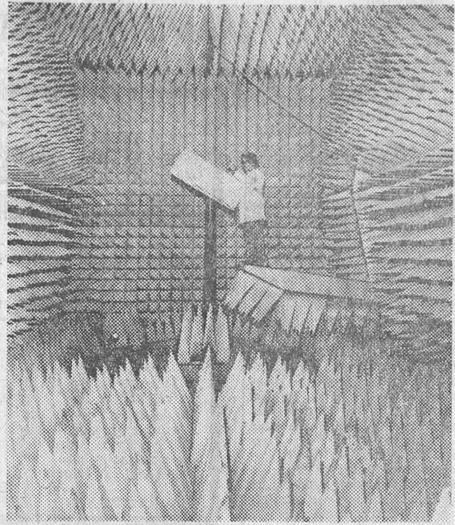
No, no se trata de eso. Es un recinto de radiaciones del «Electronic and Space System Group» de la «British Aircraft Corporation» en el que se simulan las condiciones de espacio libre mediante el empleo de un material que absorbe las radiaciones para así comprobar la exacta medida de patrones de radiación de antenas para vehículos aéreos. Curioso. — (F. F.)
