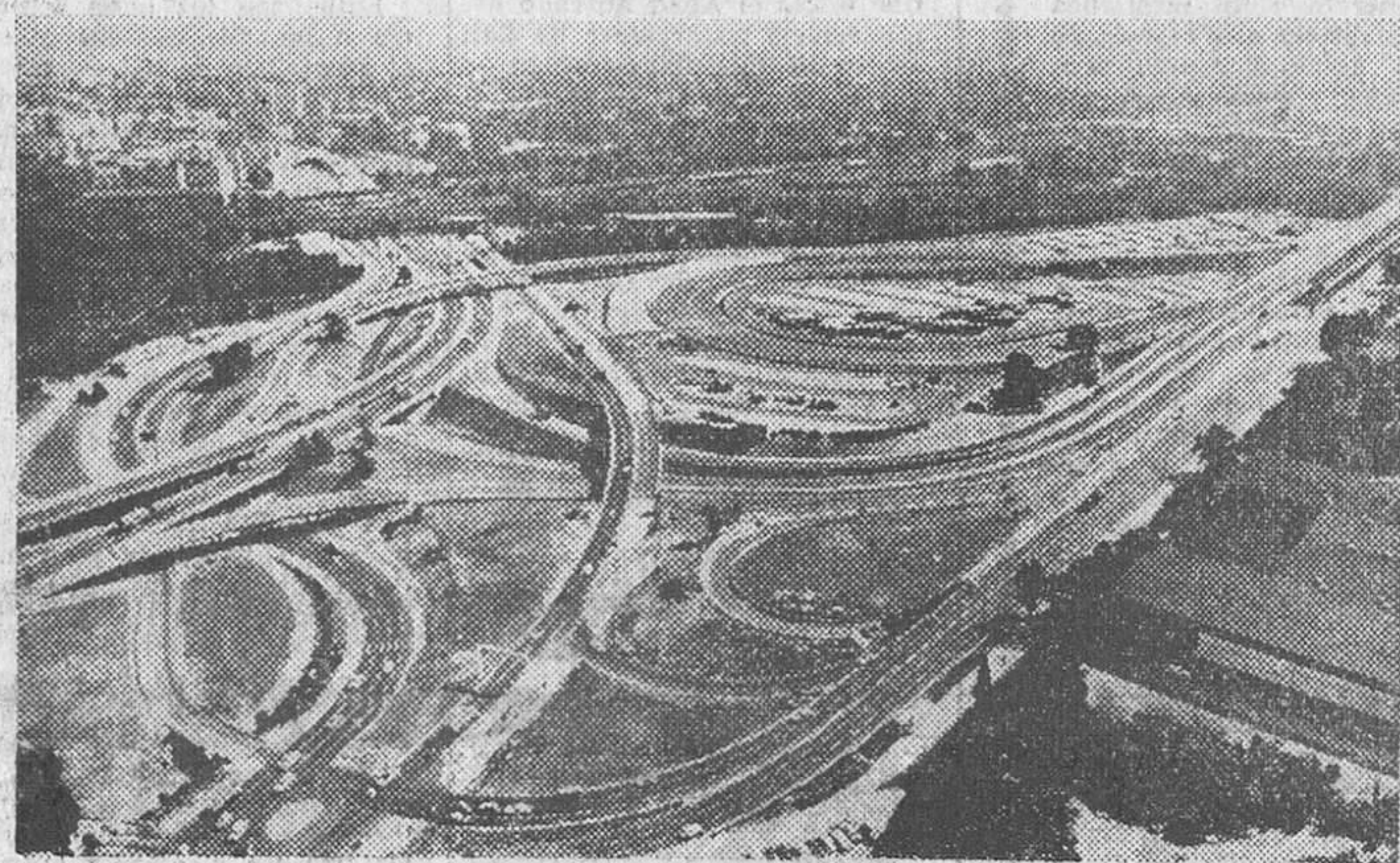
Este lío de autopistas está en pleno Berlín Oeste y se llama "Distribuidor de la AVUS" que es la ruta más frecuentada de la Alemania Federal. En 24 horas circular por aquí 76.000 automóviles. Para completar este "distribuidor" sin cruces fue necesario construir trece puentes, dos túneles, tres kilómetros de calzada y 900 metros de paredes de apoyo. — (DaD).
