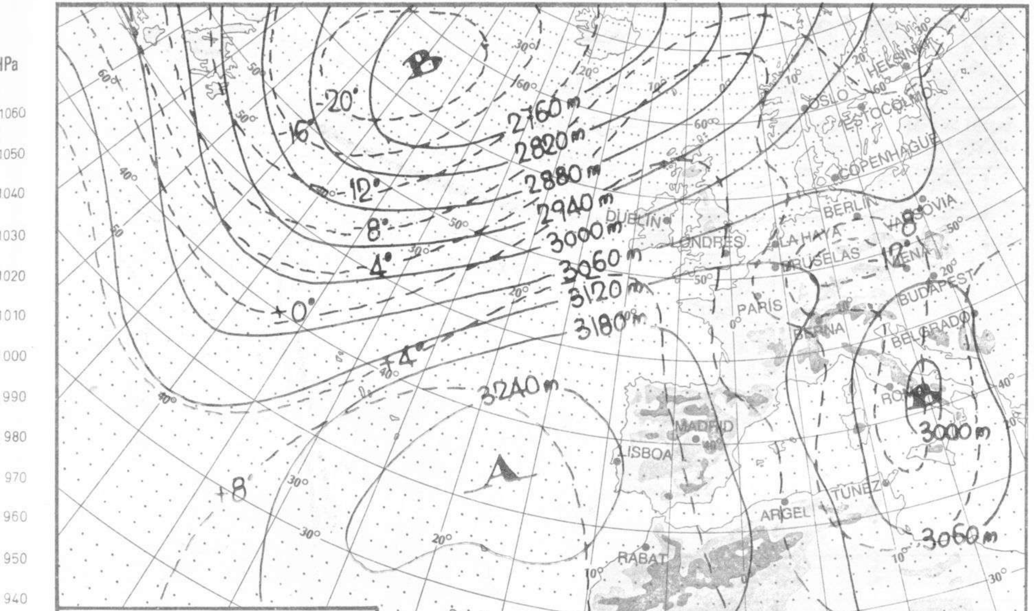
TOPOGRAFIA DE LA SUPERFICIE DE 700 HPa a 12 h. (TMG) Día 27-10-86
