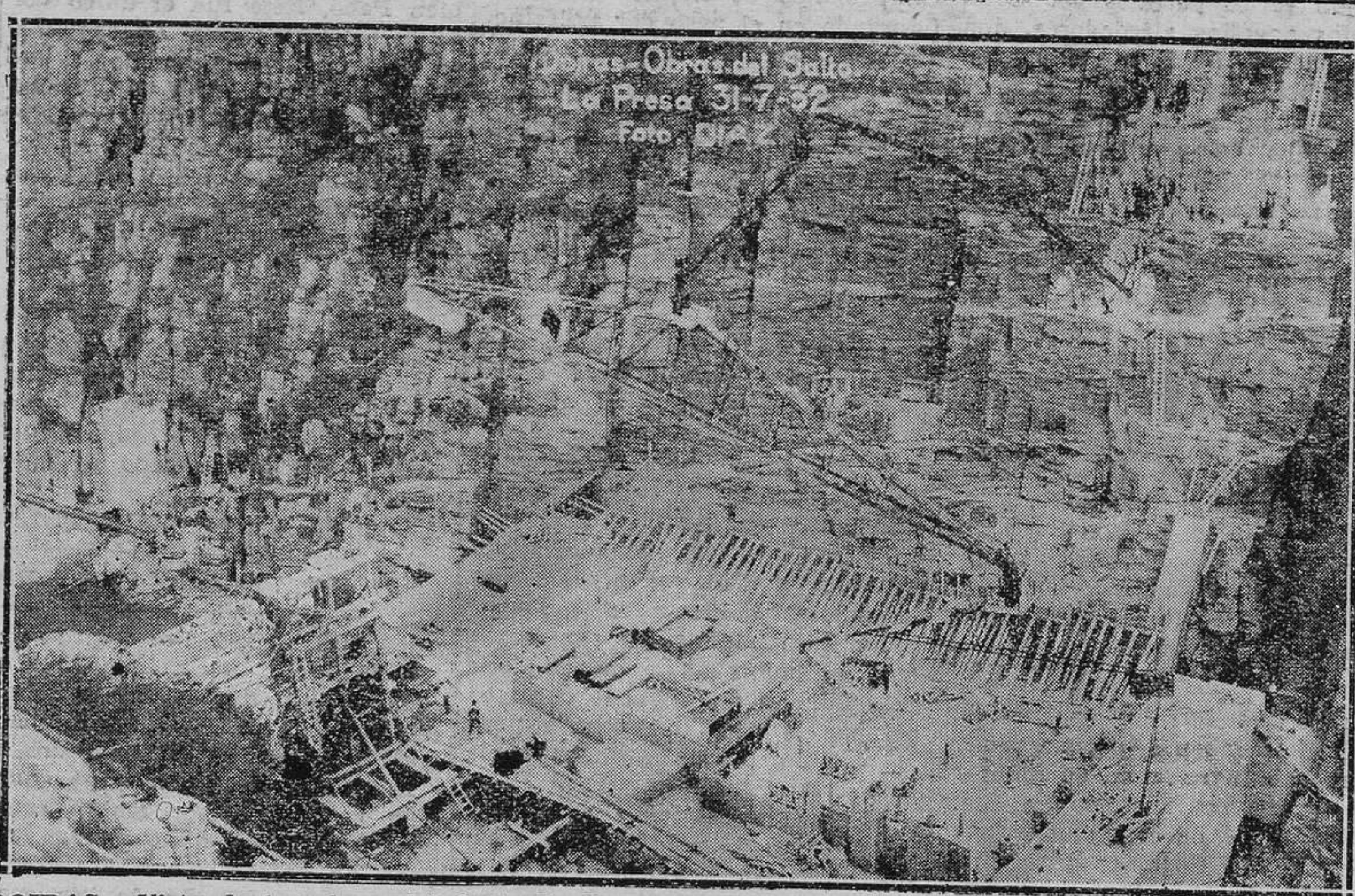
DOIRAS.—Vista de las obras del Salto La Presa, donde ocurrió el desprendimiento que sepultó a once obreros, pereciendo cinco. (Foto archivo REGION).
