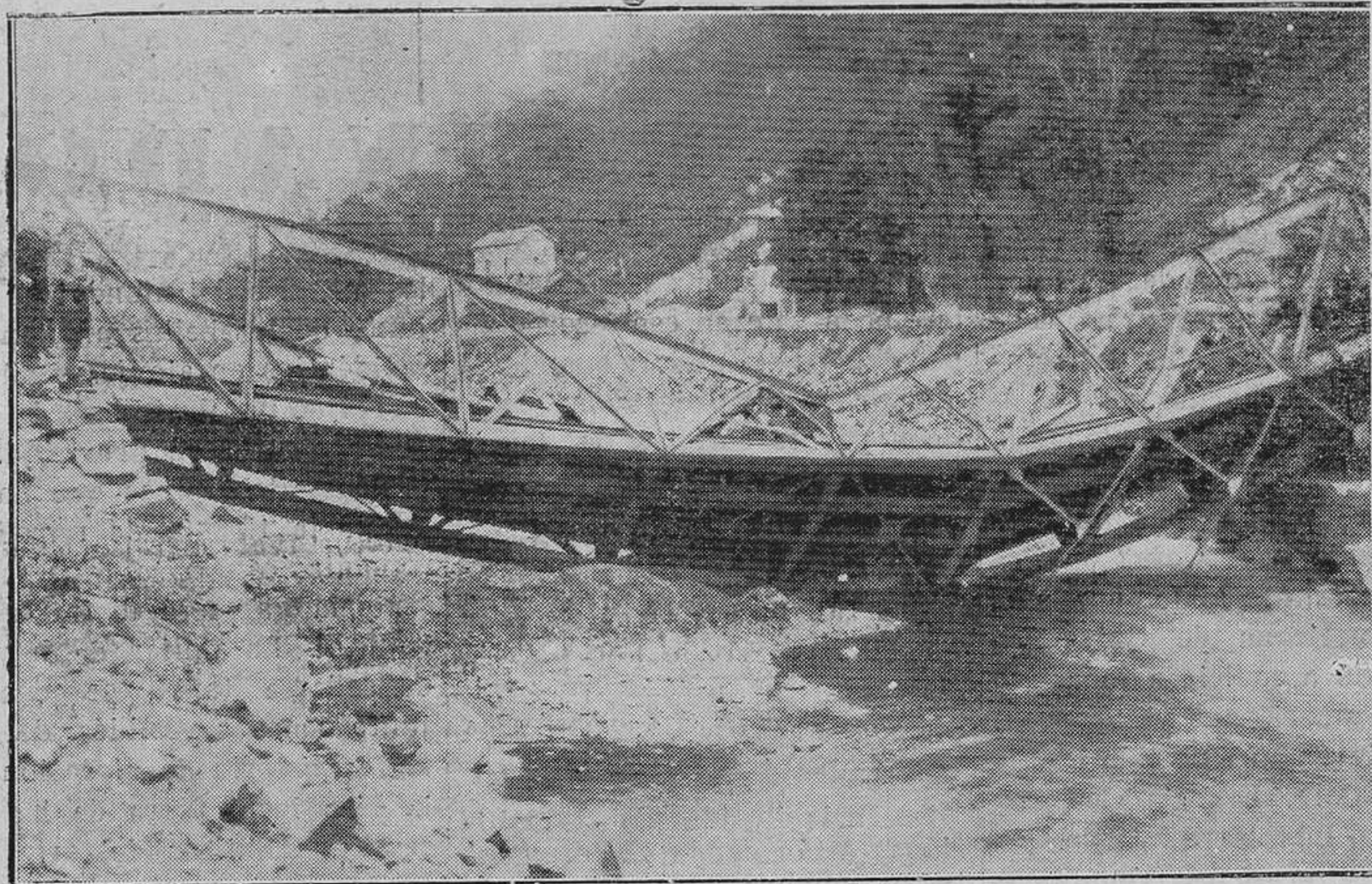
MOREDA.-Estado en que quedó el puente y material ferroviario, por hundimiento del primero, de la S. I. A. (Foto Tuero)
