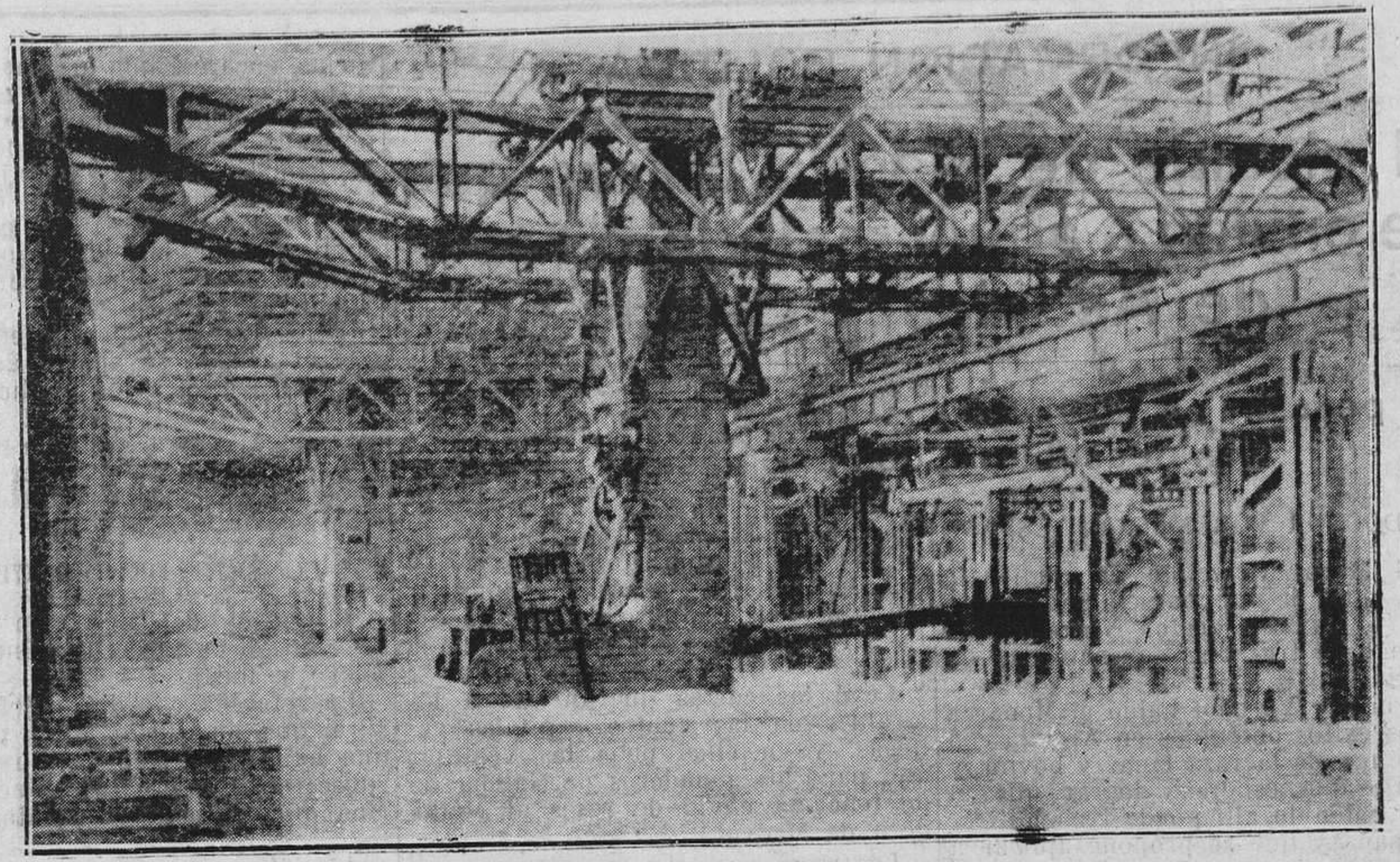
Puente rotatorio, cargado para horno Martín. [Peso 2.500 kilogramos].
