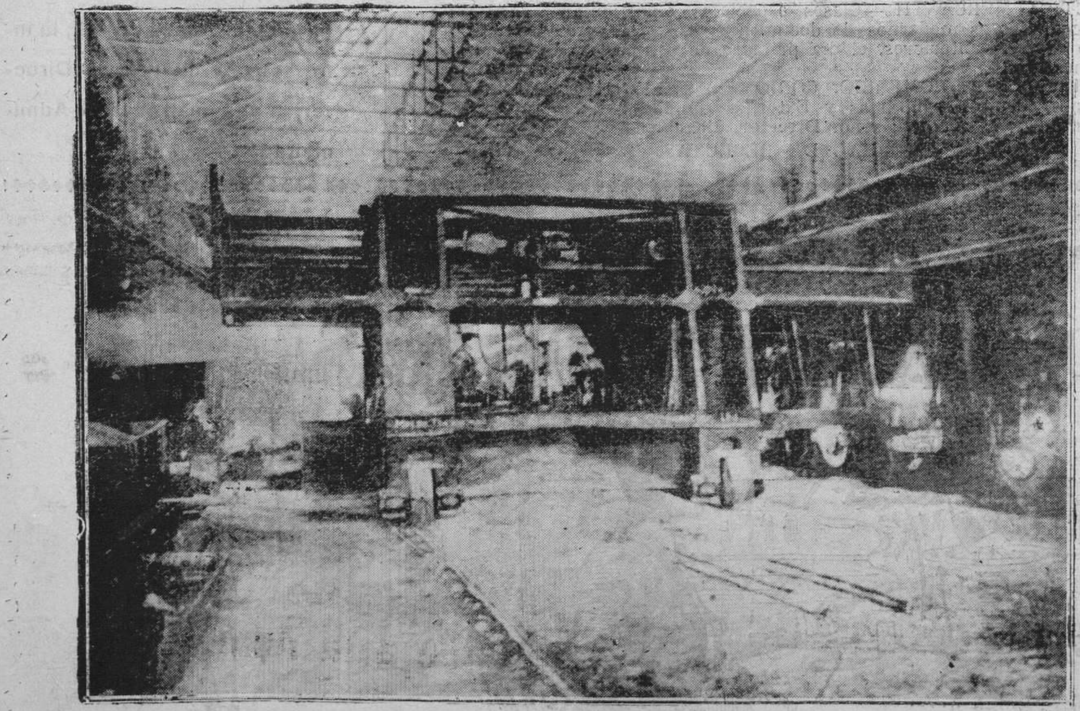
Cargador de acero, tipo Hanf, sistema Wellman, montado sobre carro que permite el rápido transporte de lingotes incandescentes.
