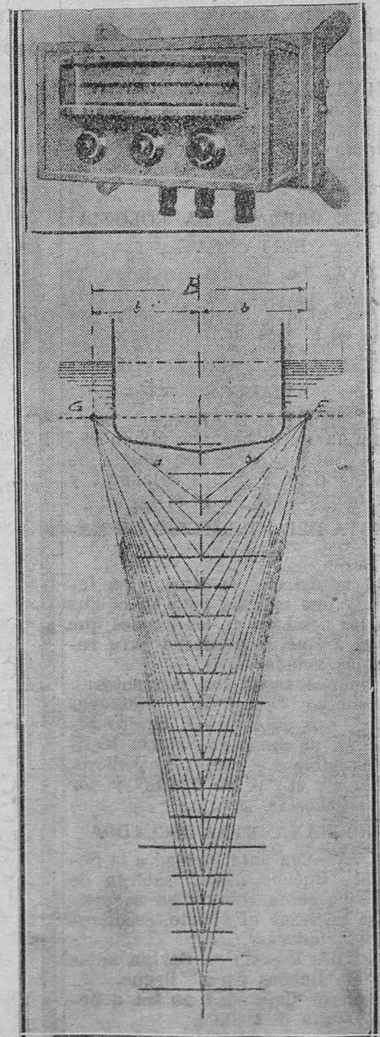
LA PROFUNDIDAD DEL MAR MEDIDA POR EL ECO.-Al estallar el cartucho, E, el sonido se refleja en el fondo del mar, y se obtiene la reproducción del eco en el aparato receptor, G, colocado en la otra borda del buque, B. Las ondas, S, se reflejan en la vertical situada a igual distancia de E y G.-Aguja indicadora de las profundidades.
