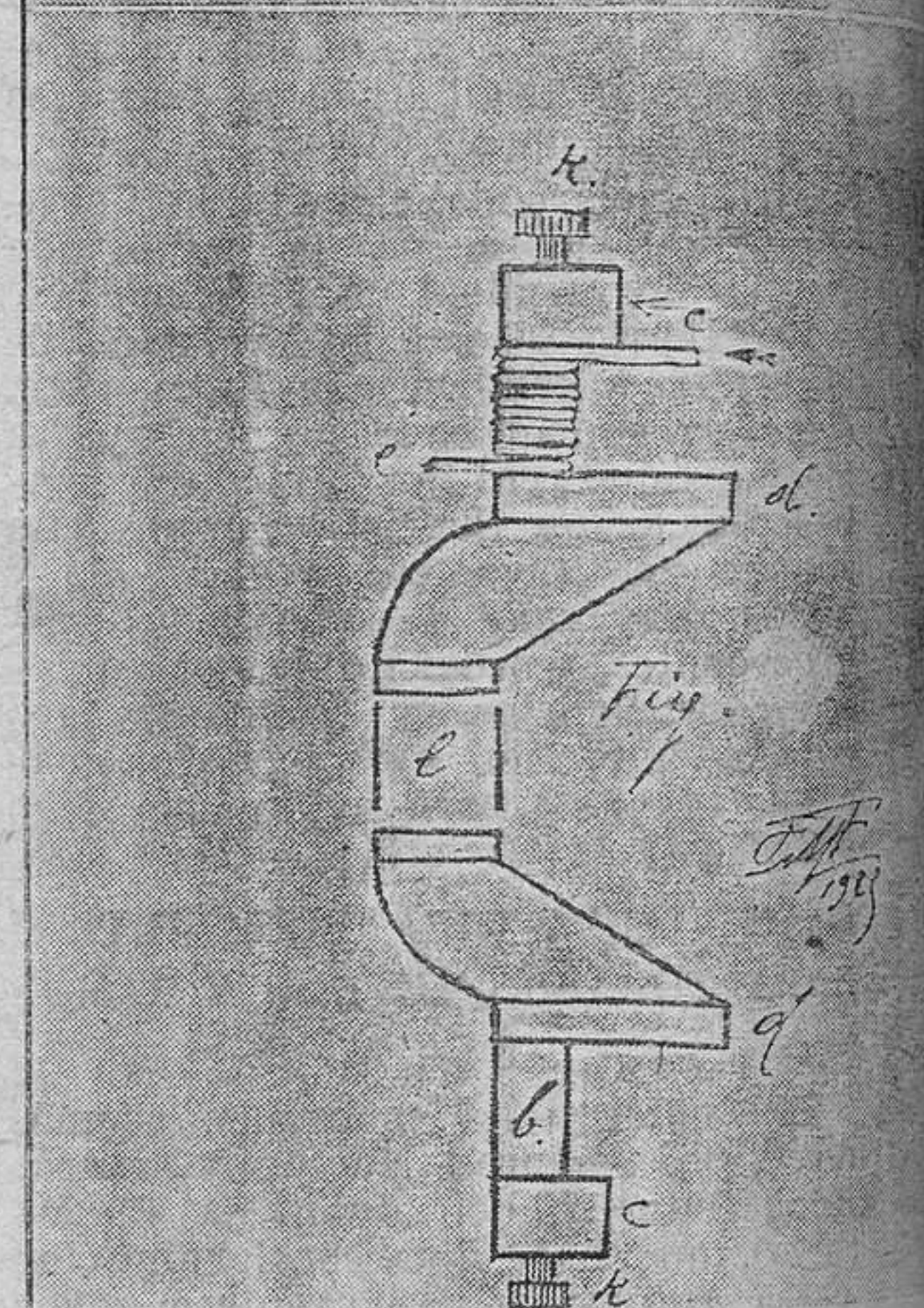
Corte transversal del inductor, b. cilindro de los inductores; d. idem; e. circuito de excitación longitudinal de uno de los órganos inductores; b. bobinado de los inductores; e. circuito de excitación; d. anillos de los inductores, como c; k. tornillos de sujeción.
