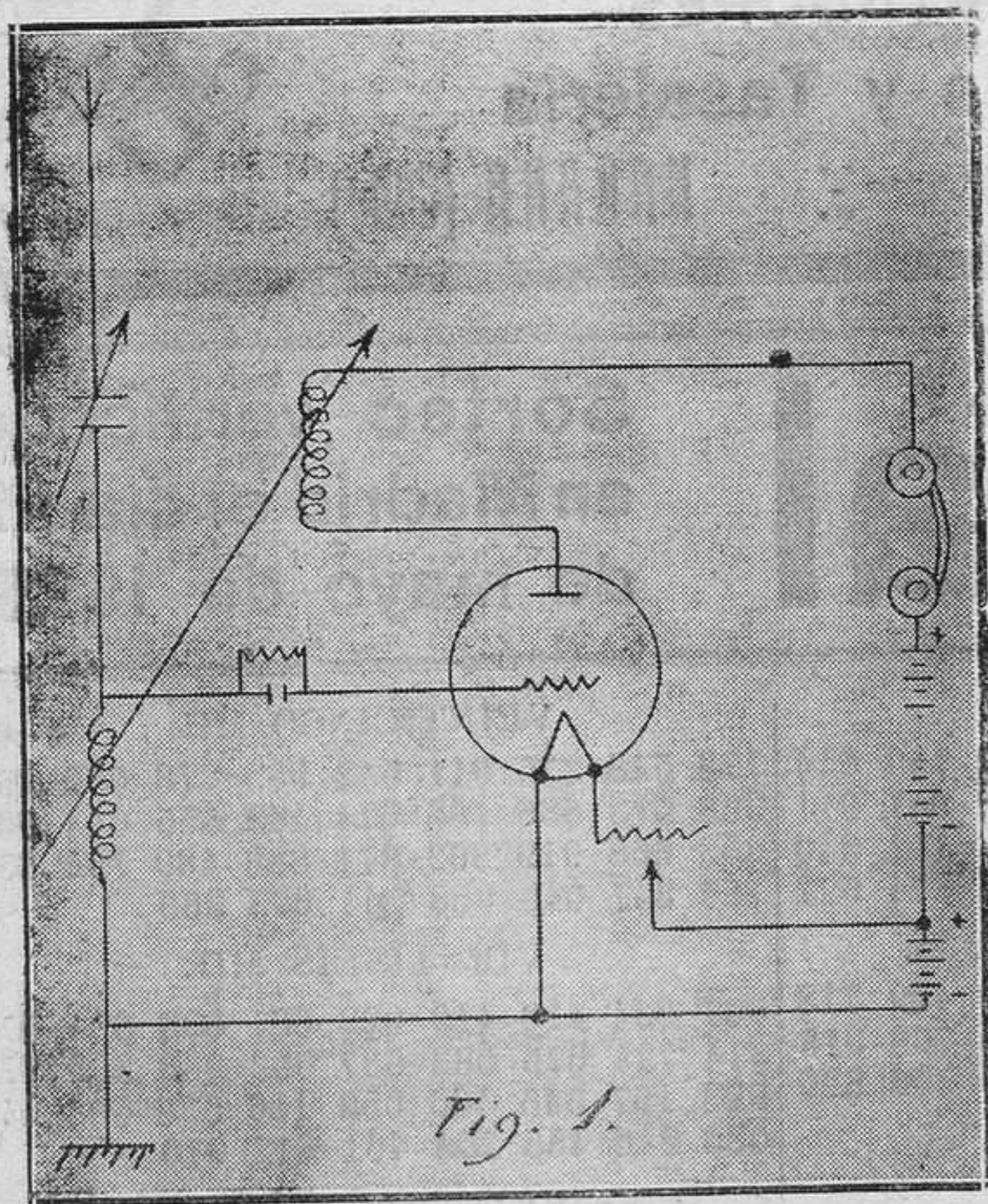
Lámpara detectora.
