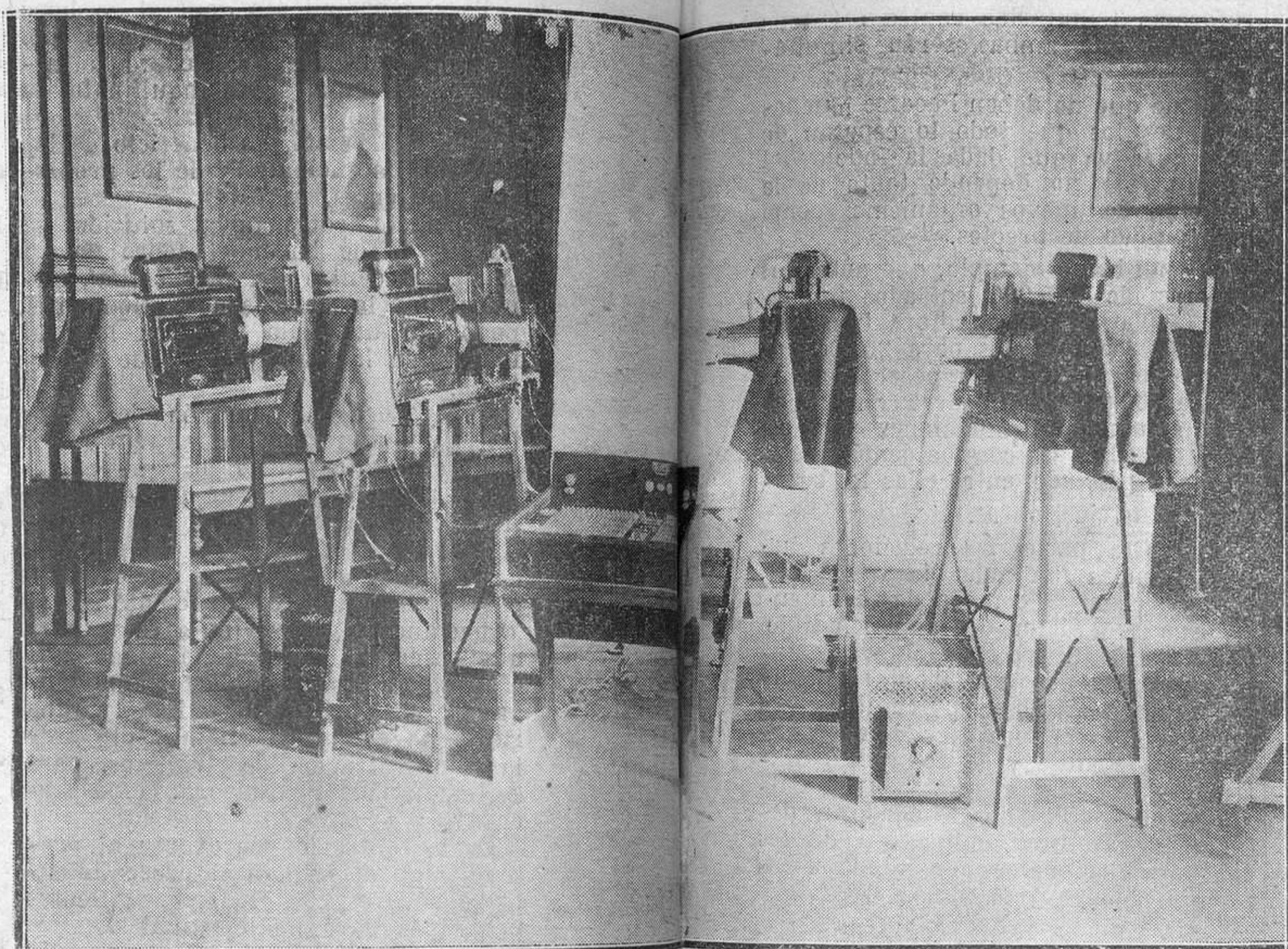
Las cuatro grandes piezas del piano de luz de color, vistas desde el lado del pianista. (Foto Vidal)
