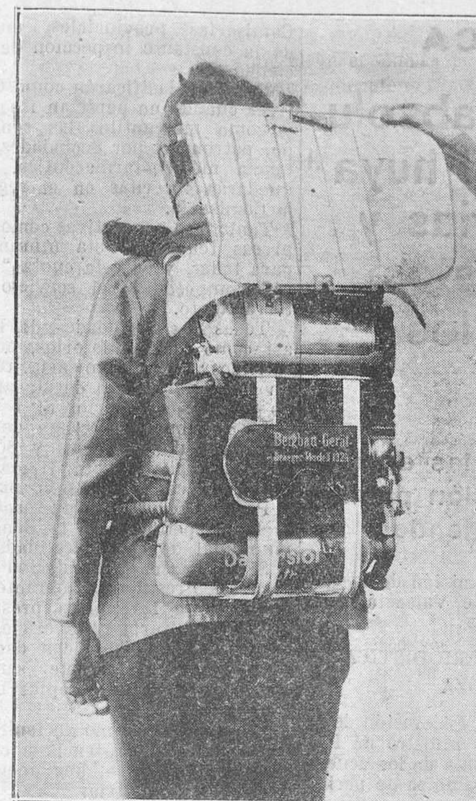
El nuevo equipo de salvación en minas, visto por detrás. (Foto Vidal)
