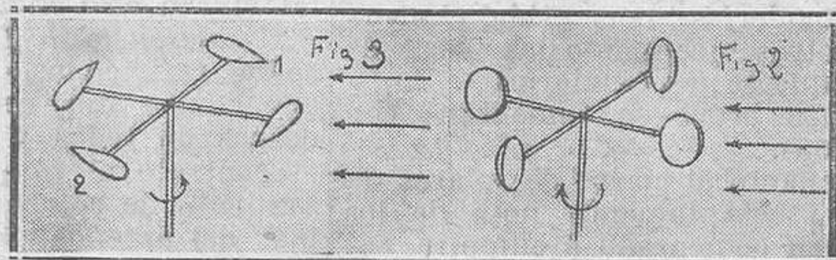
Fig. 2.-Principio de un autogiro.--Fig. 3.--Otra forma de autogiro.
