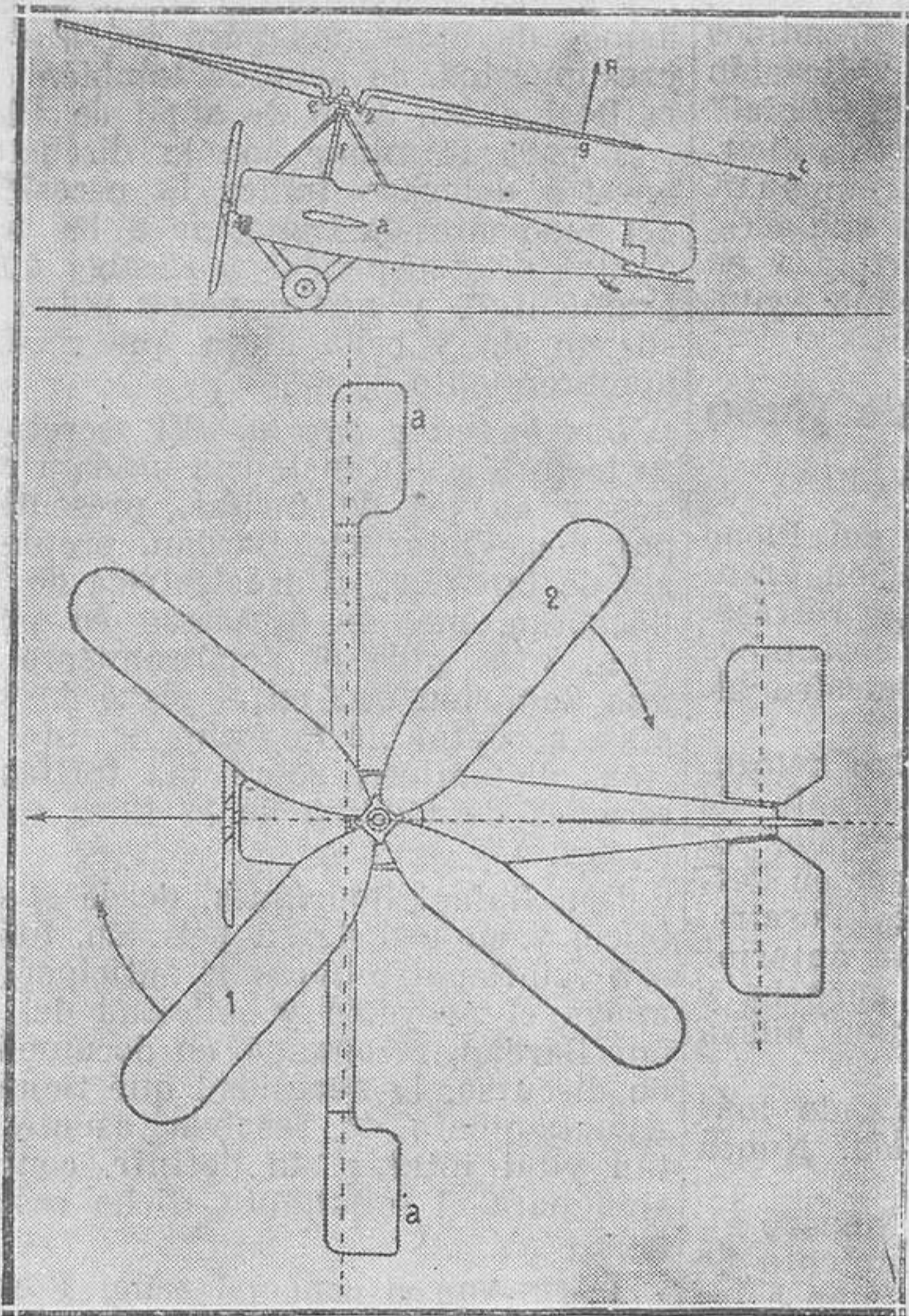
Figura 1.-Explicación del vuelo y de la estabilidad del "Autogiro".
