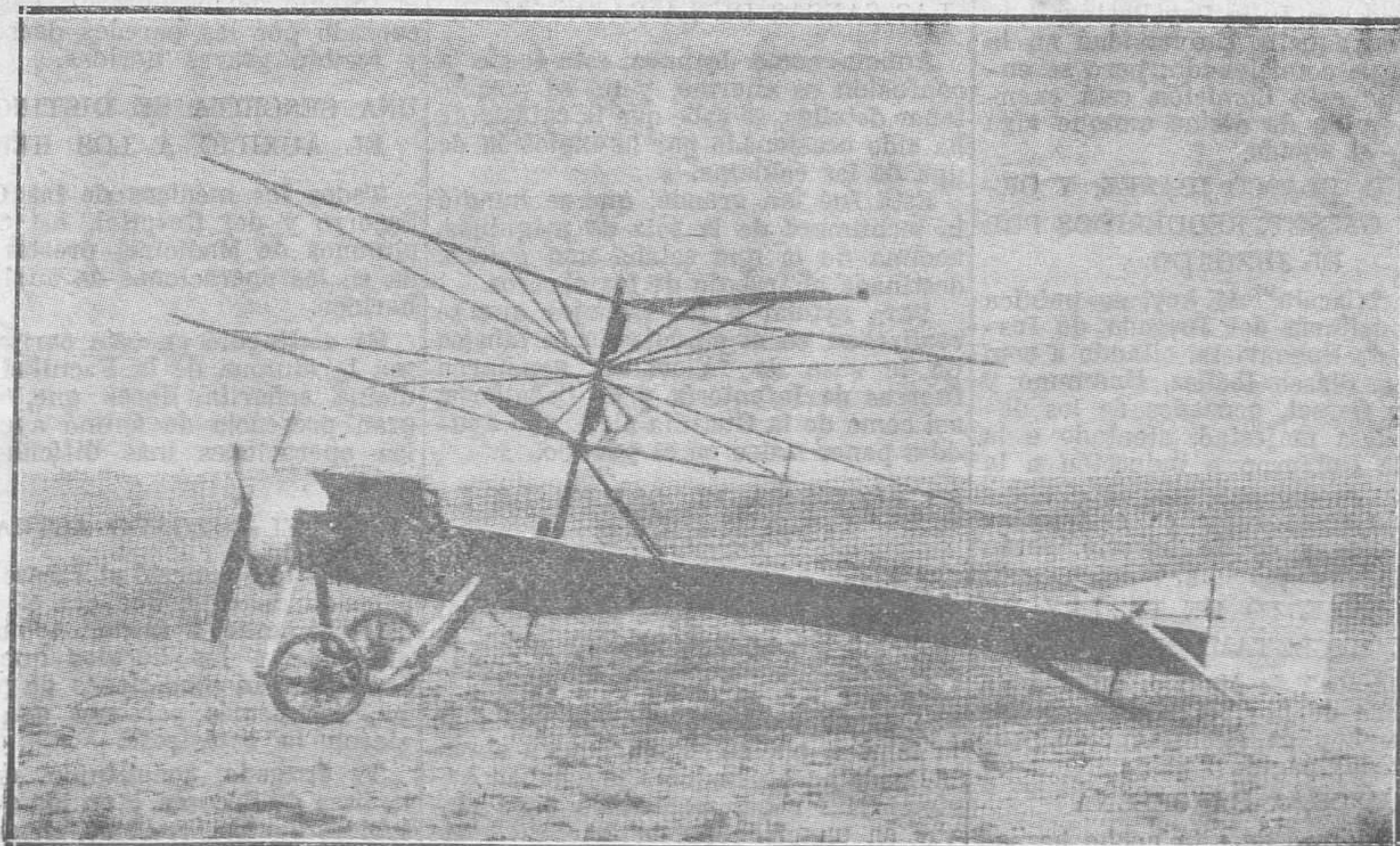
El primer aparato del ingeniero señor Cierva, llevaba dos hélices, a fin de compensar la simetría señalada en la leyenda de la figura 1.
