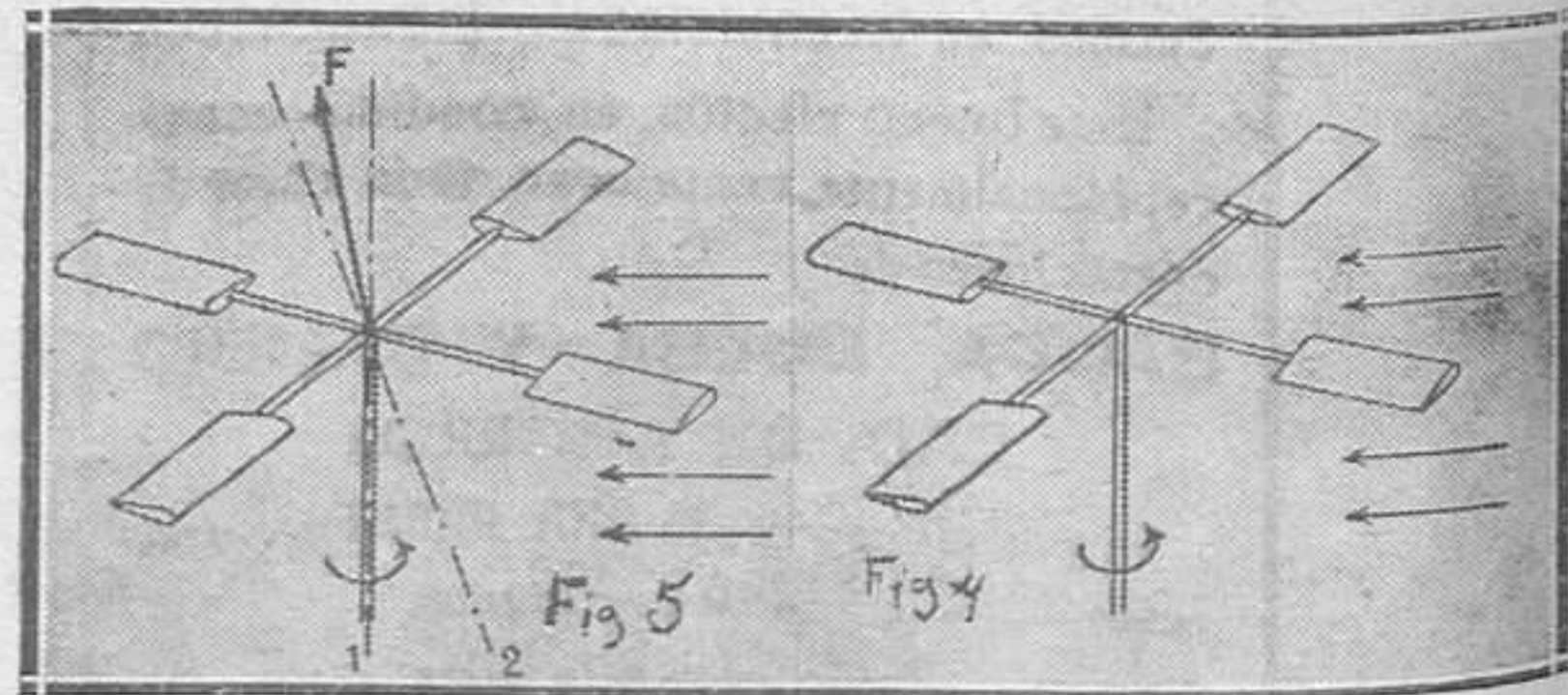
Fig. 4.-Autogiro de alas. Estas tienen una sección disimétrica y análoga a la de los cuerpos pisciformes. Gira el conjunto en el sentido de la flecha.-- Fig. 5.-Principio del "Autogiro": El eje vertical, posición 1, permite girar al aparato bajo la influencia del viento. Si se inclina el eje hasta la posición 2, hace una fuerza, F, dirigida hacia arriba. Esta fuerza es superior a la que puede desarrollar en el mismo sentido un ala de aeroplano.
