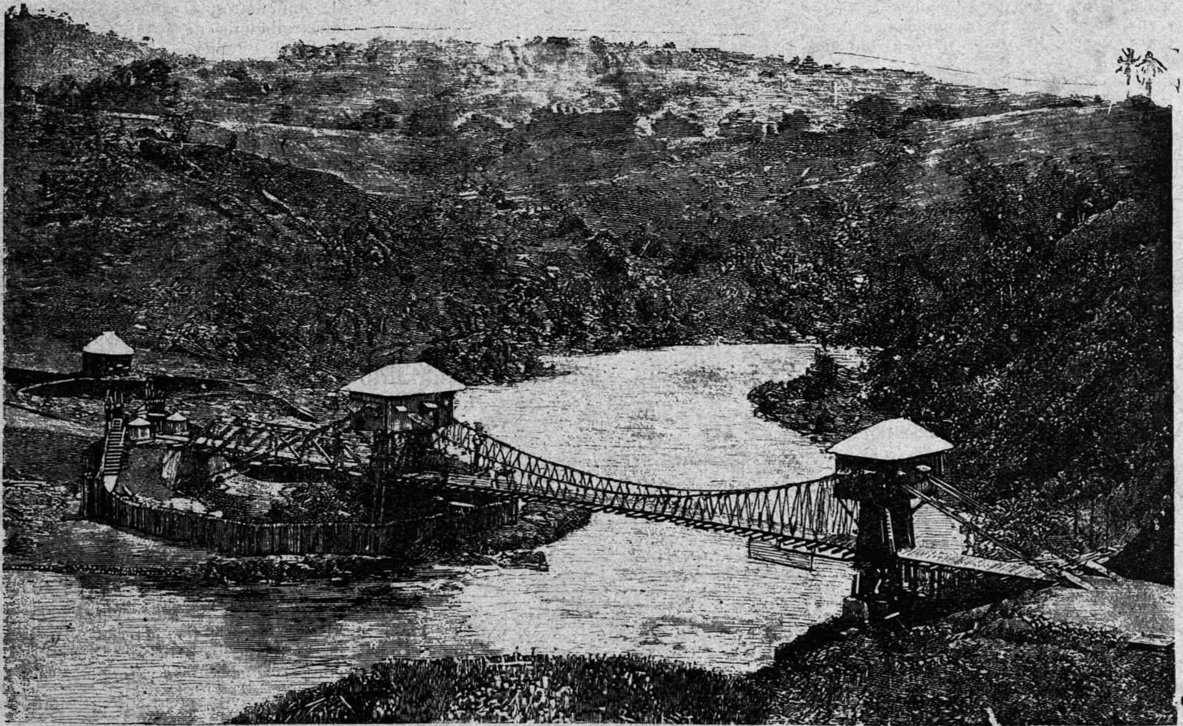
EJÉRCITO ESPAÑOL EN FILIPINAS—LA CAMPAÑA DE MINDANAO—Puente colgante sobre el rio Agus, construido por los ingenieros militares españoles en solo 15 dias, bajo la dirección del comandante D. Rafael Ravena
