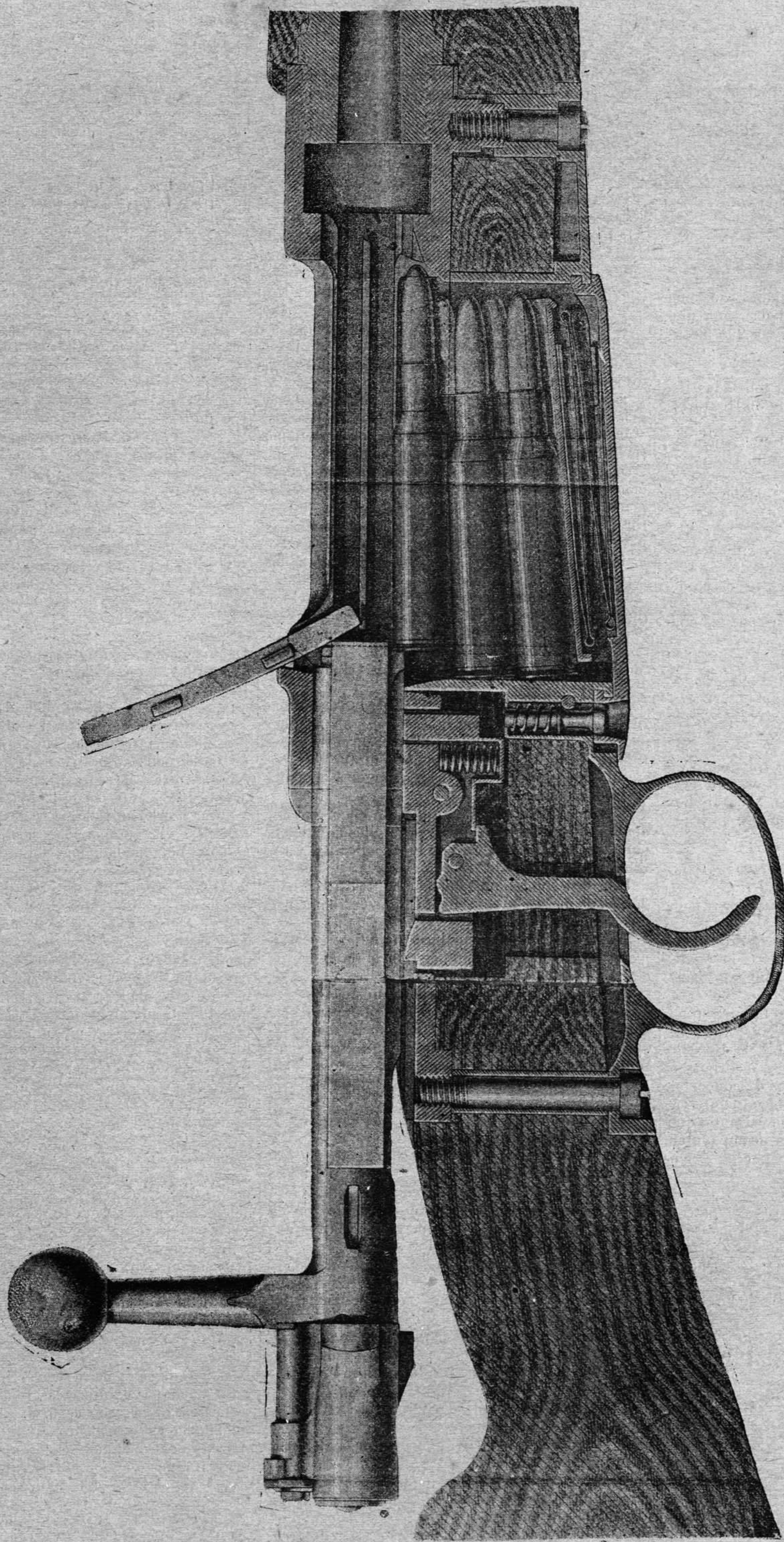
FUSIL MAUSER ESPAÑOL—MODELO 1893, CALIBRE 7 MM., ADOPTADO PARA LOS EJÉRCITOS ESPAÑOL, CHILENO, BRASILEÑO Y ALEMÁN
