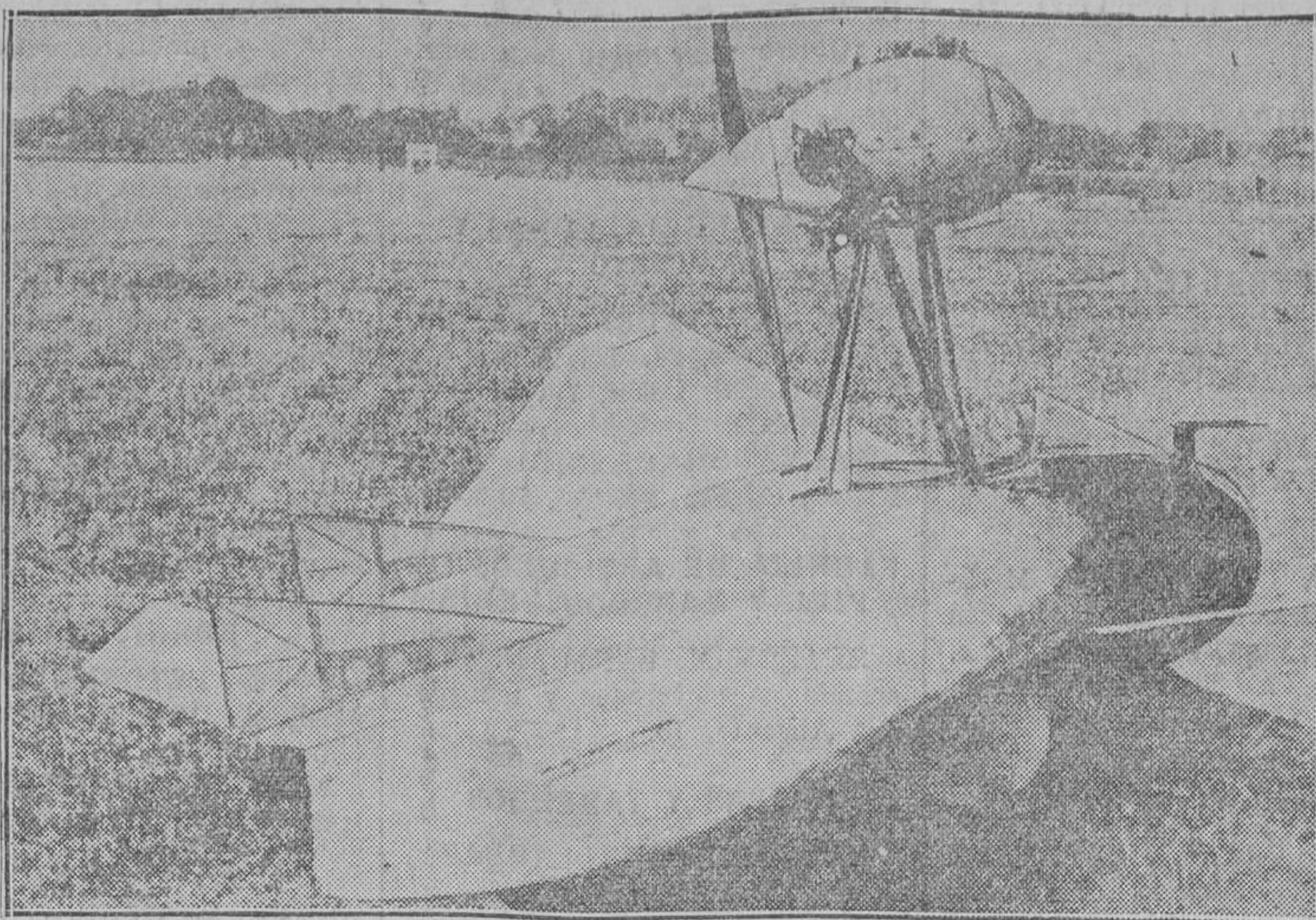
Este modelo abreviado de aeroplano, que tiene por objeto reducir la resistencia del viento y facilitar vuelos con un motor de 32 caballos, está listo para los ensayos en el aeródromo de Coudron, cerca a París
