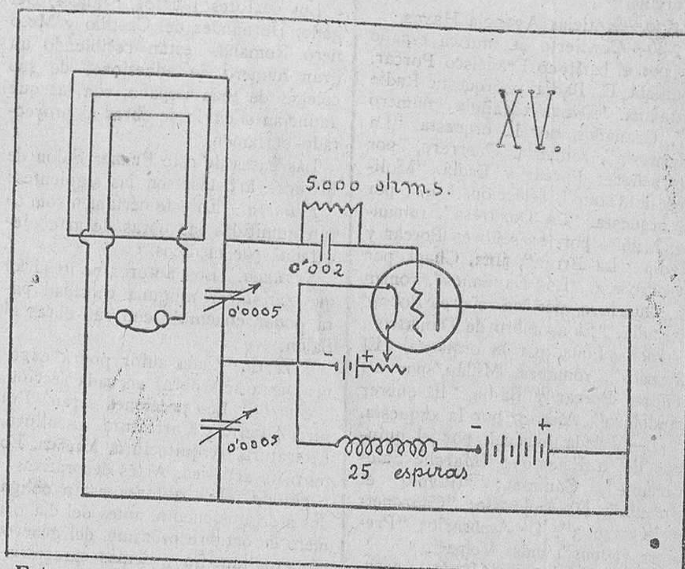
Este aparato no funciona. Sin tocar el circuito de placa, hay que subsanar dos errores. Una vez subsanados, FUNCIONA, y es tan potente que puede escucharse desde muy lejos.
