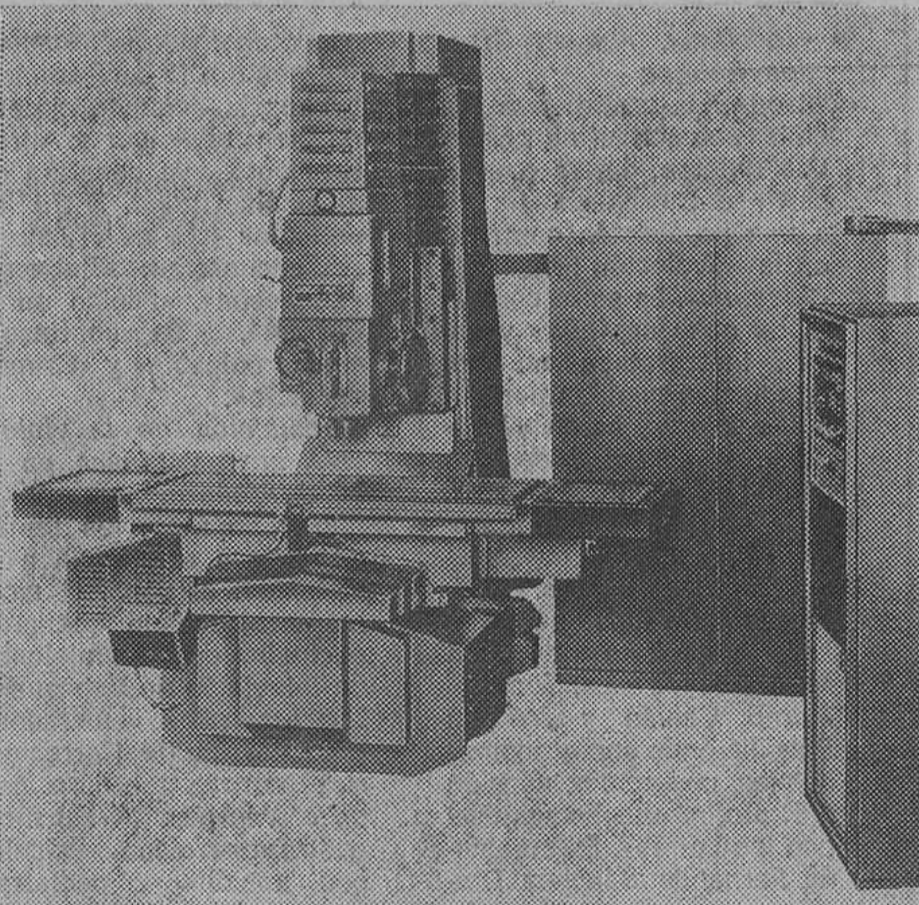
1 - Modelo ANAK-MATIC-12 CN con control numérico NC-3000 (AURKI)
