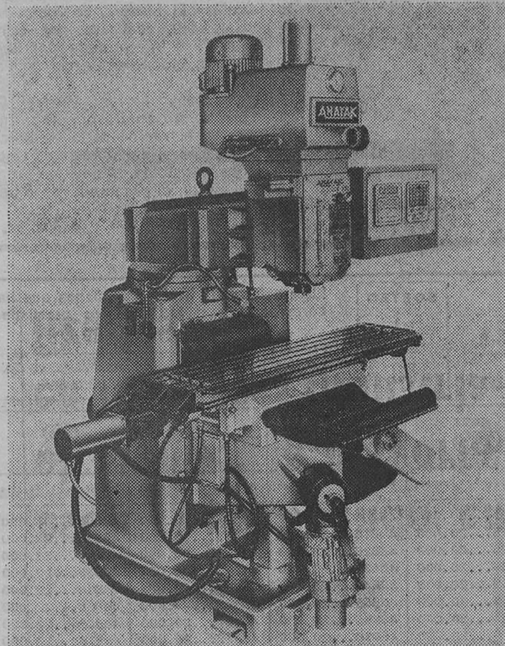
3 - Modelo CNC-1000 con control numérico MATE-M (SIEMENS)
