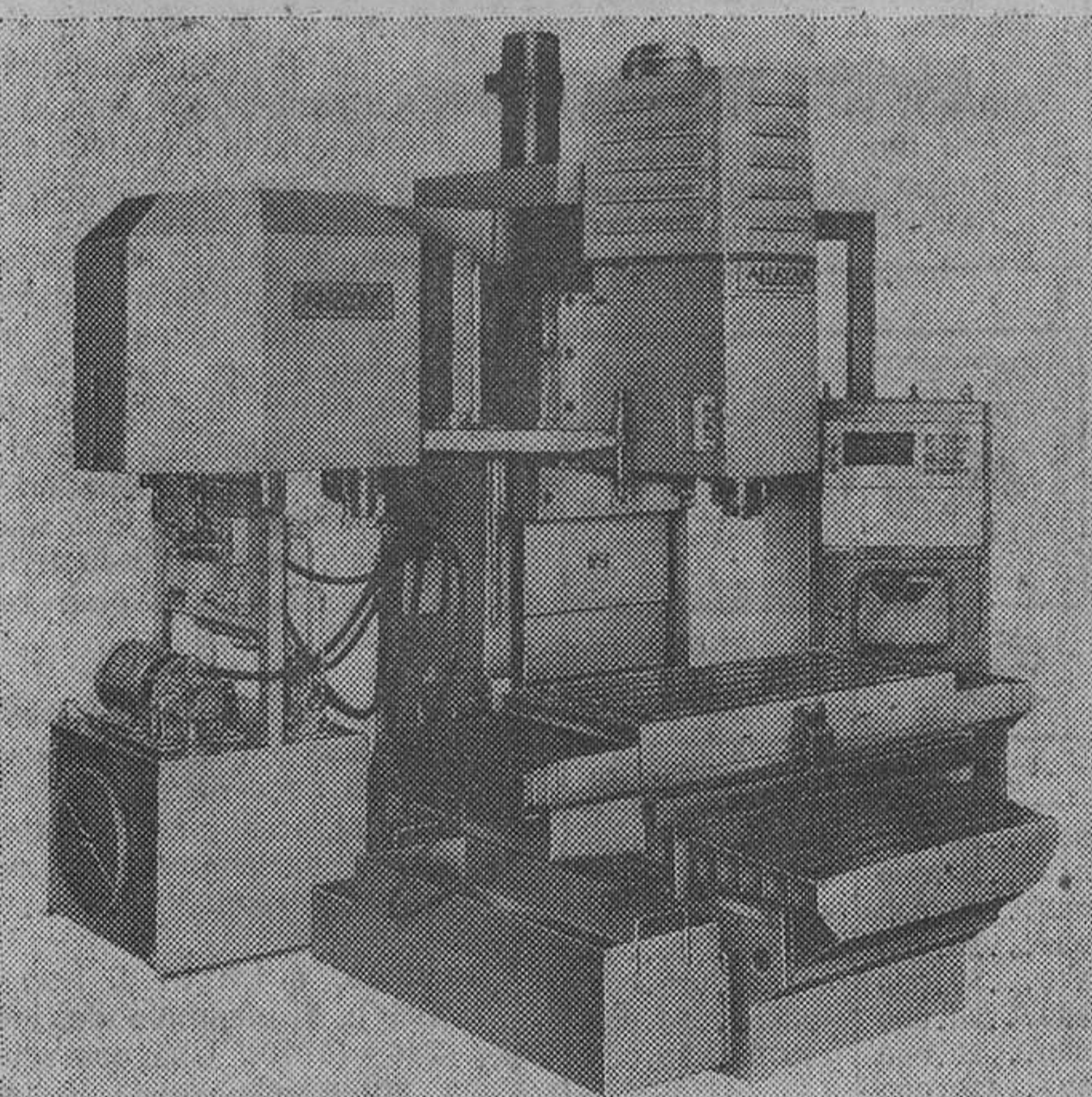
2 - Modelo ANAK-MATIC-10 CNC con control numérico Sinumerik-6 M (SIEMENS)
