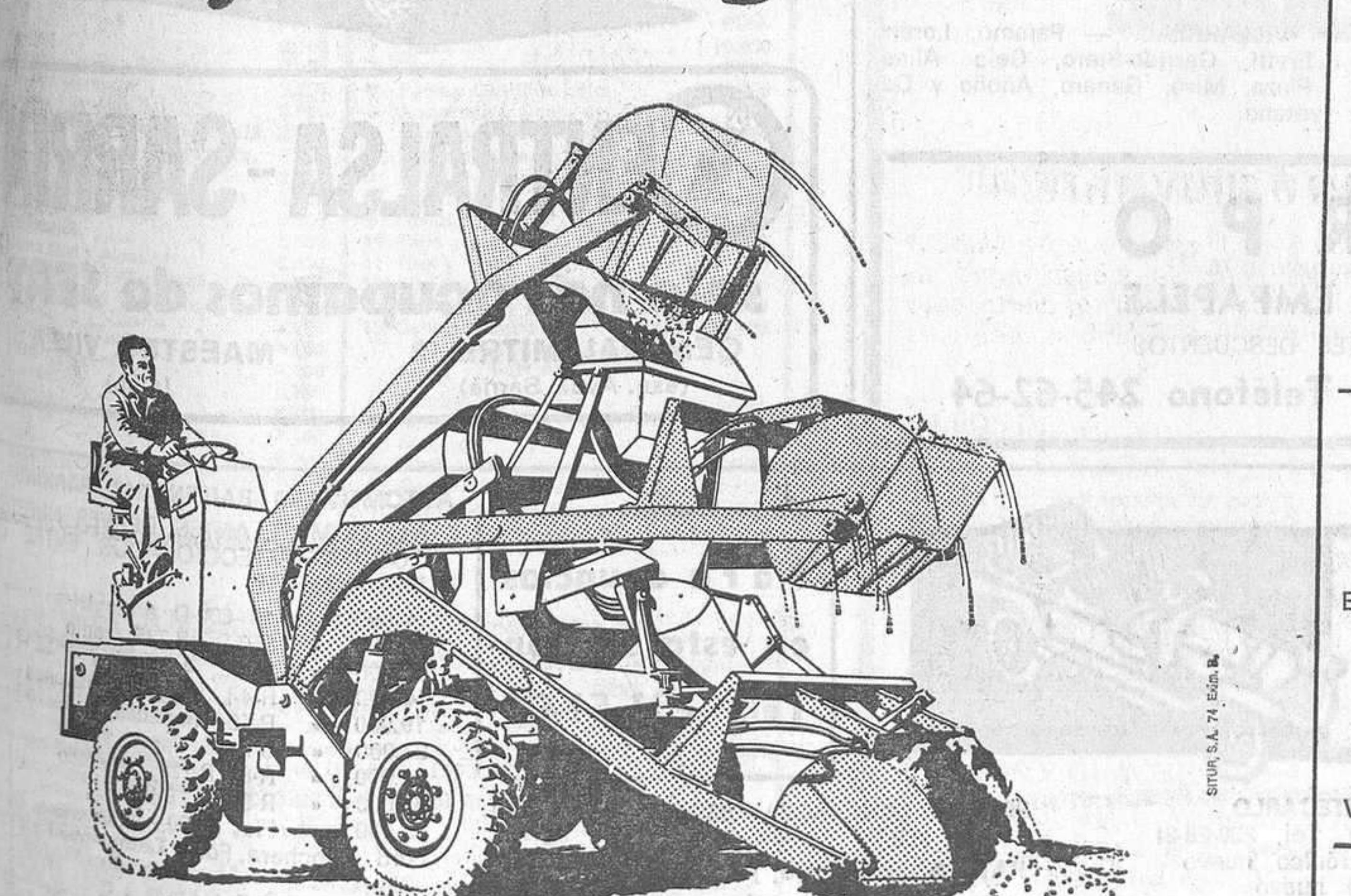
La autohormigonera CARMAN significa autonomía y rentabilidad; se autocarga, dosifica, amasa, transporta y descarga ganando tiempo y eliminando equipo auxiliar y mano de obra.
