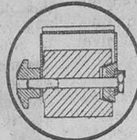
dispositivo de freno de las ruedas delanteras
