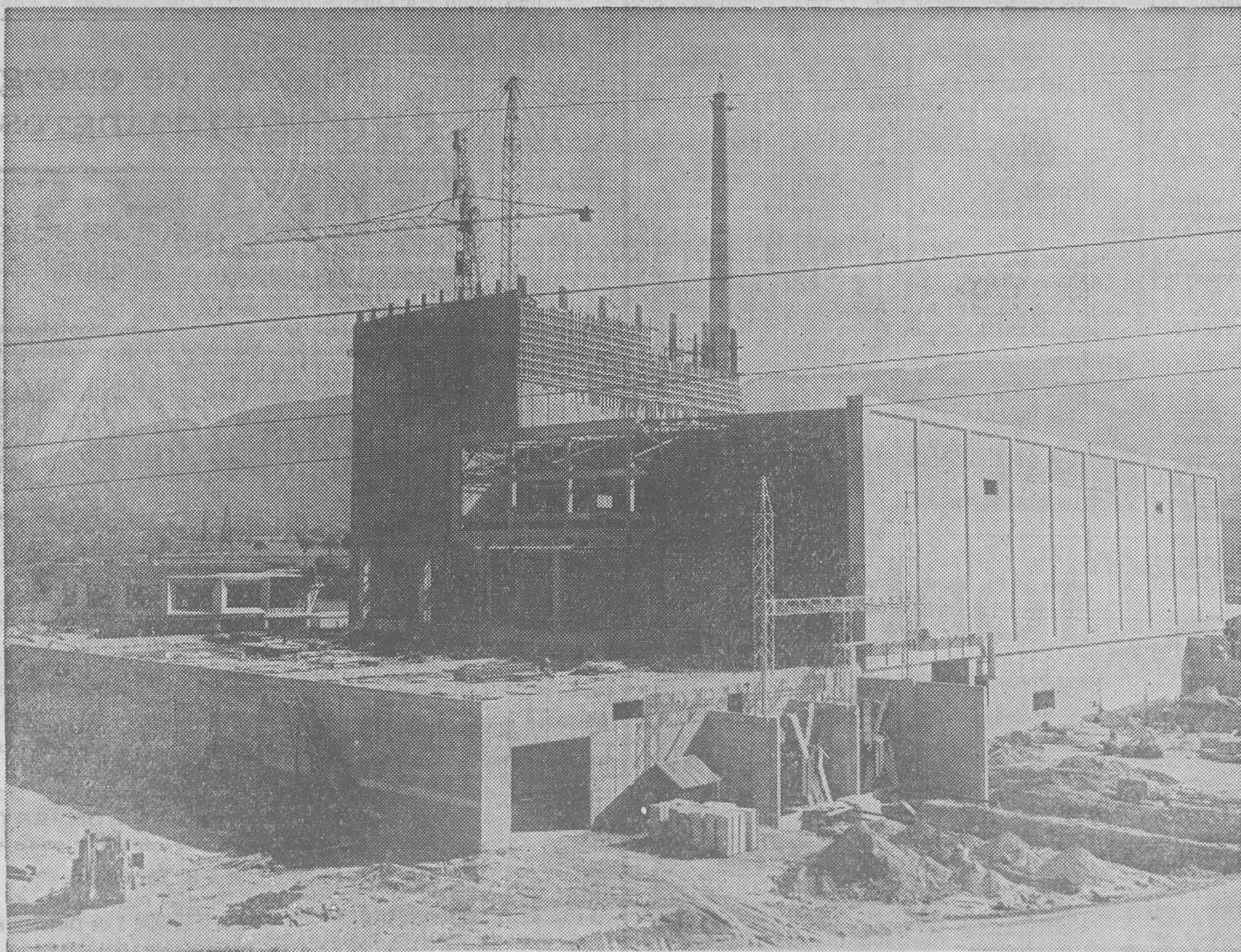
Central Nuclear de Santa María de Garoña — Burgos
