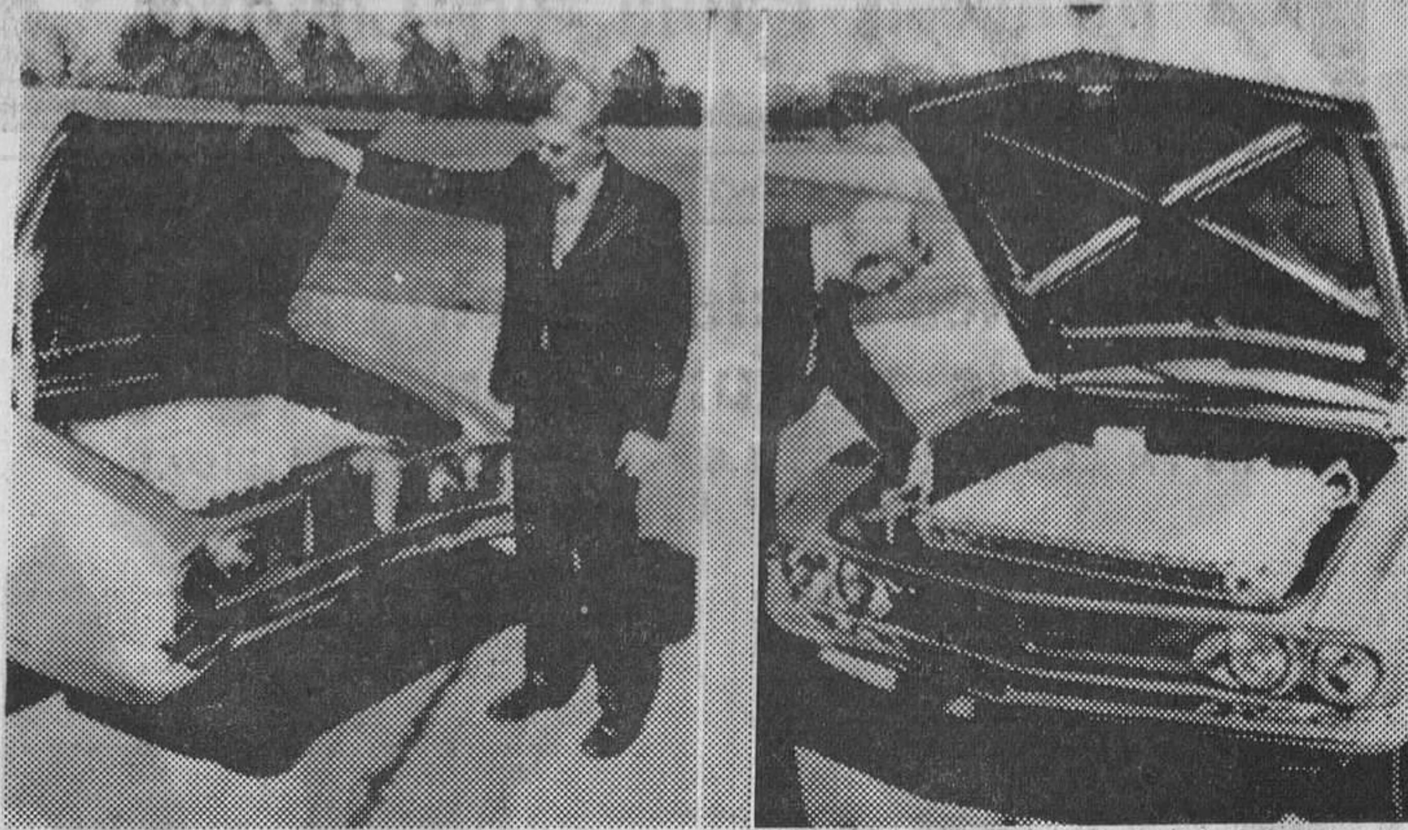
Detroit. — Vista de la parte anterior y posterior de sendos modelos experimentales del «Corvaire II», contruidos por la «General Motors», mostrando las baterías de zinc plateado que accionan eléctricamente los vehículos. — (Telefoto Cifra.)
