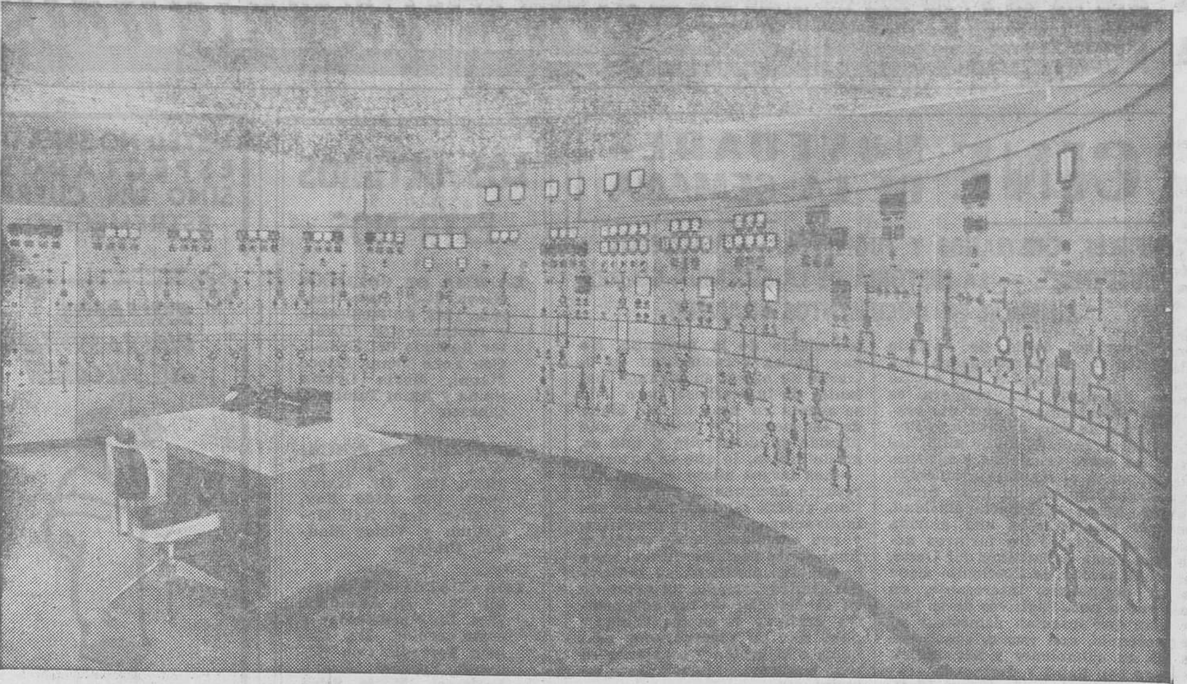
La automatización sigue un ritmo creciente en las modernas actividades. Esta es la subestación que Hidroeléctrica de Cataluña tiene instalada en San Andrés. Un solo hombre controla desde su mesa el esquema sinóptico que aparece en esa sala de cuadros de mando y gobierna las instalaciones de 110 KV y 25 KV. Así se regula con toda facilidad y sin el riesgo de otros tiempos
