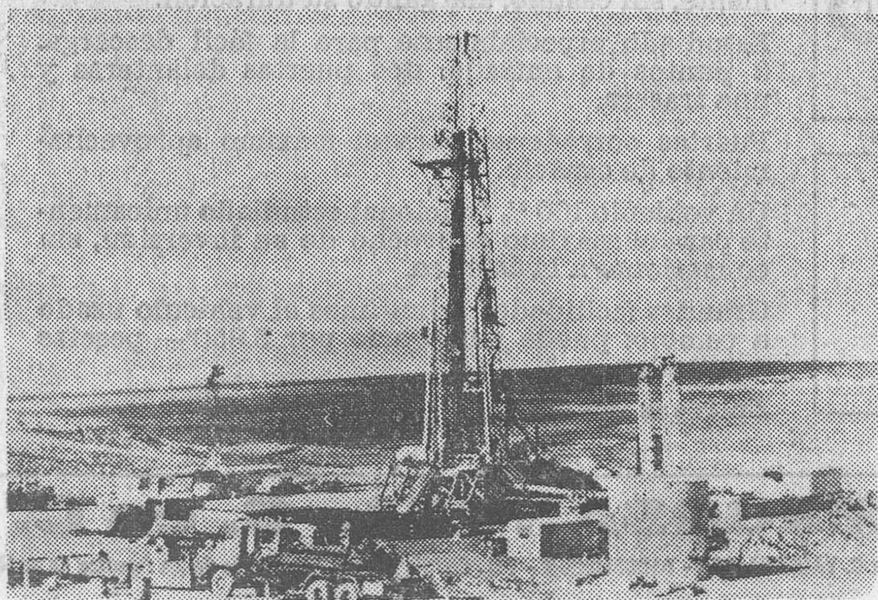
Burgos. — En el yacimiento petrolífero de La Lora se han iniciado los trabajos de sondeo que señalan la apertura del pozo «Ayoluengo III», que aparece en la presente nota gráfica. Es propósito de las compañías prospectoras imprimir la mayor celeridad a dichos trabajos, con el fin de aprovechar al máximo el tiempo, antes de que lleguen los rigores invernales (Foto Cifra)
