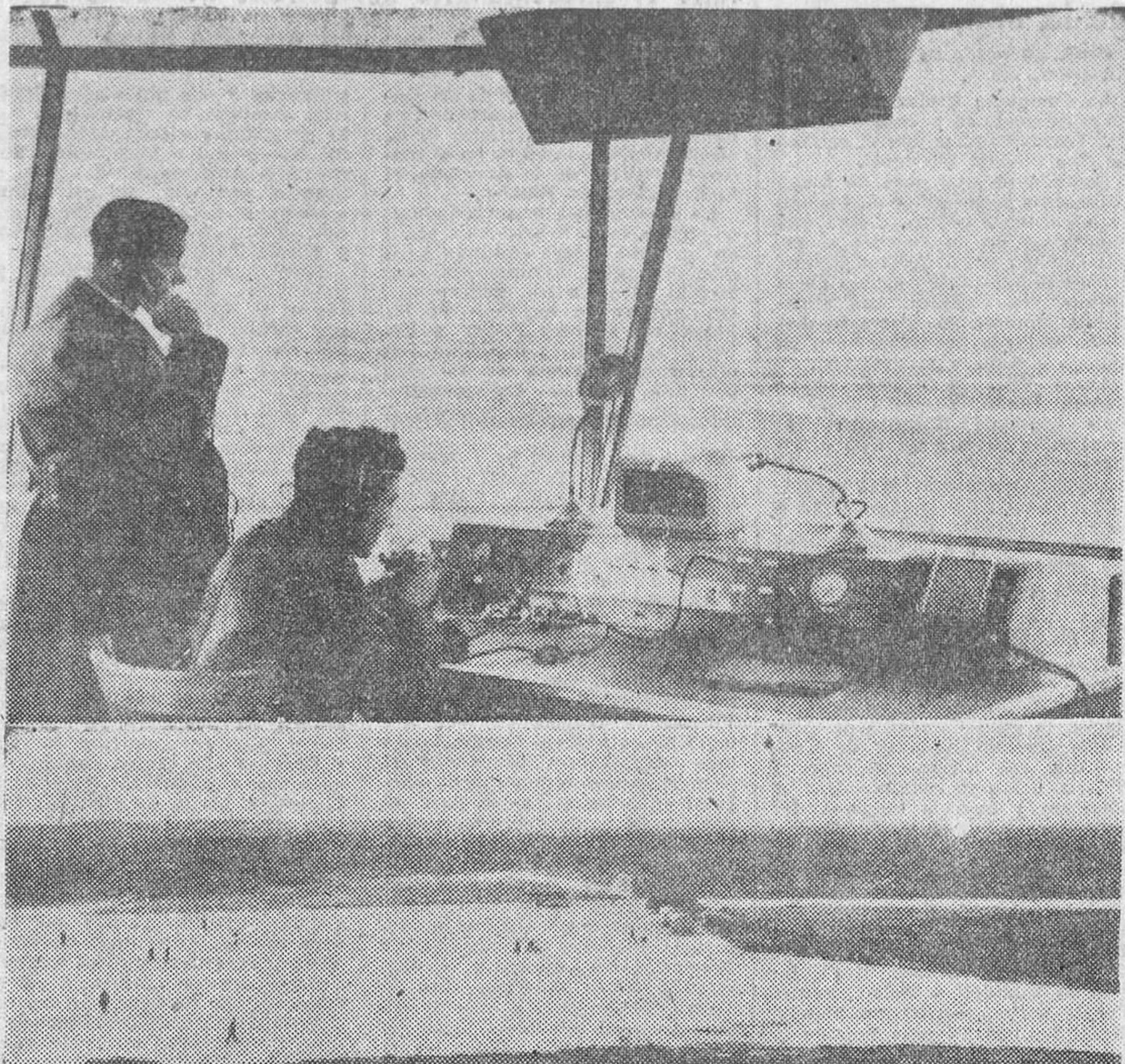
Aspecto interior de la torre de mandos del campo de aviación de Talavera la Real, donde se ha instalado la primera escuela española de pilotos para aparatos de propulsión. — Debajo, vista parcial de las pistas. — (Fotos Cifra.)
