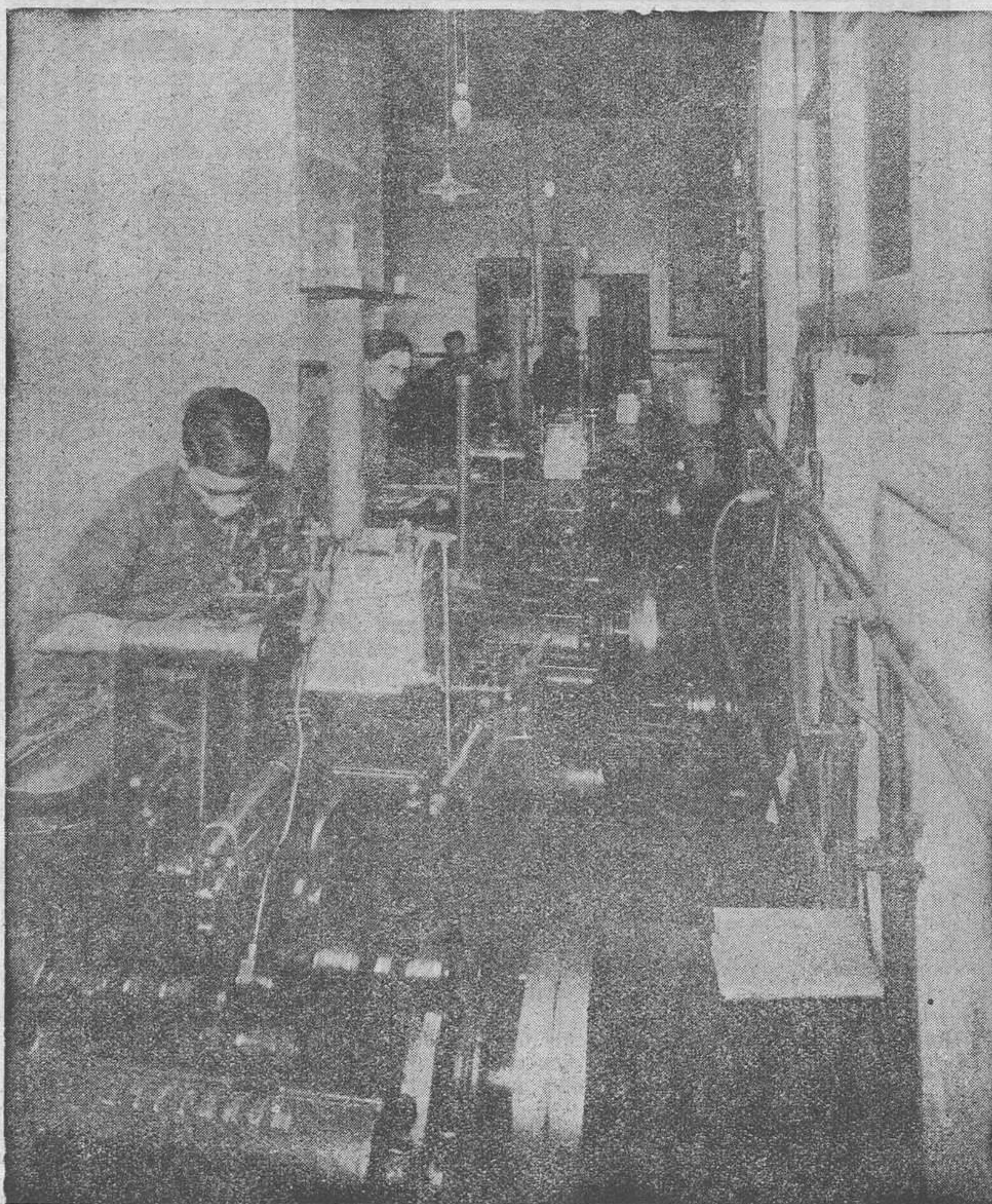
Sección de Monotypes (teclados)
