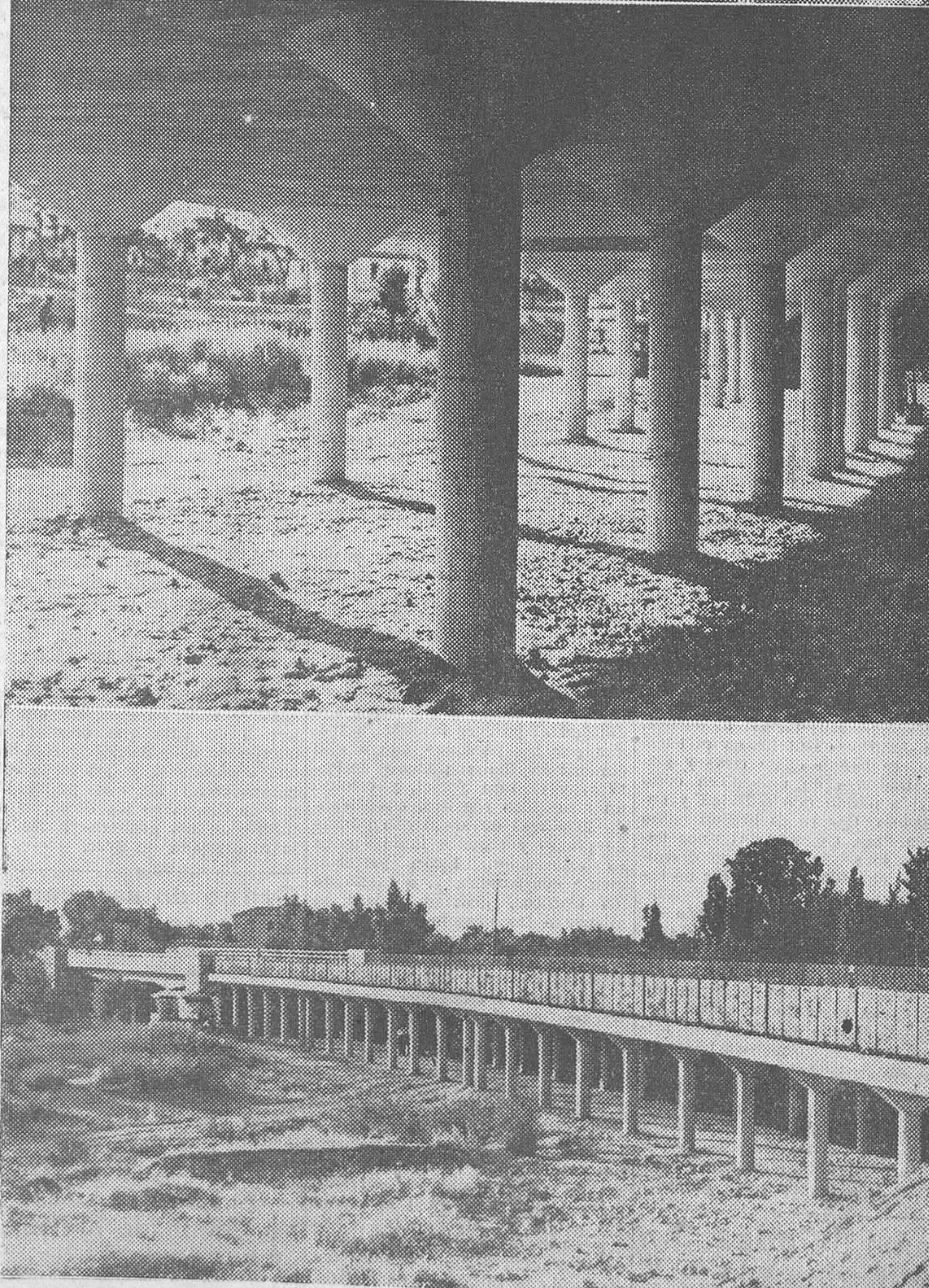
El ministro de Obras públicas inaugurando, ayer tarde, el puente que une Puerta de Hierro con la Cuesta de las Perdices, de cuya construcción dan idea las dos fotografías posteriores (Fotos Alfonso.)
