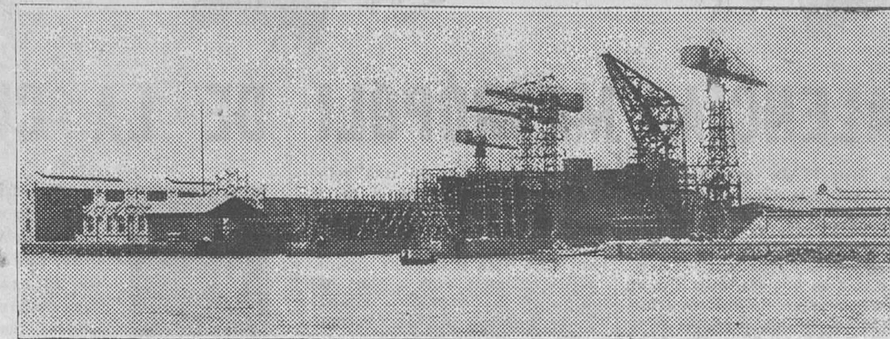
UNA VISTA GENERAL DE LOS ASTILLEROS DE LA UNION NAVAL DE LEVANTE, EN VALENCIA.—LAS GRUAS-TORRES SON, COMO SI DIJERAMOS, EL DECORADO TEATRAL DE ESTA INMENSA FACTORIA
