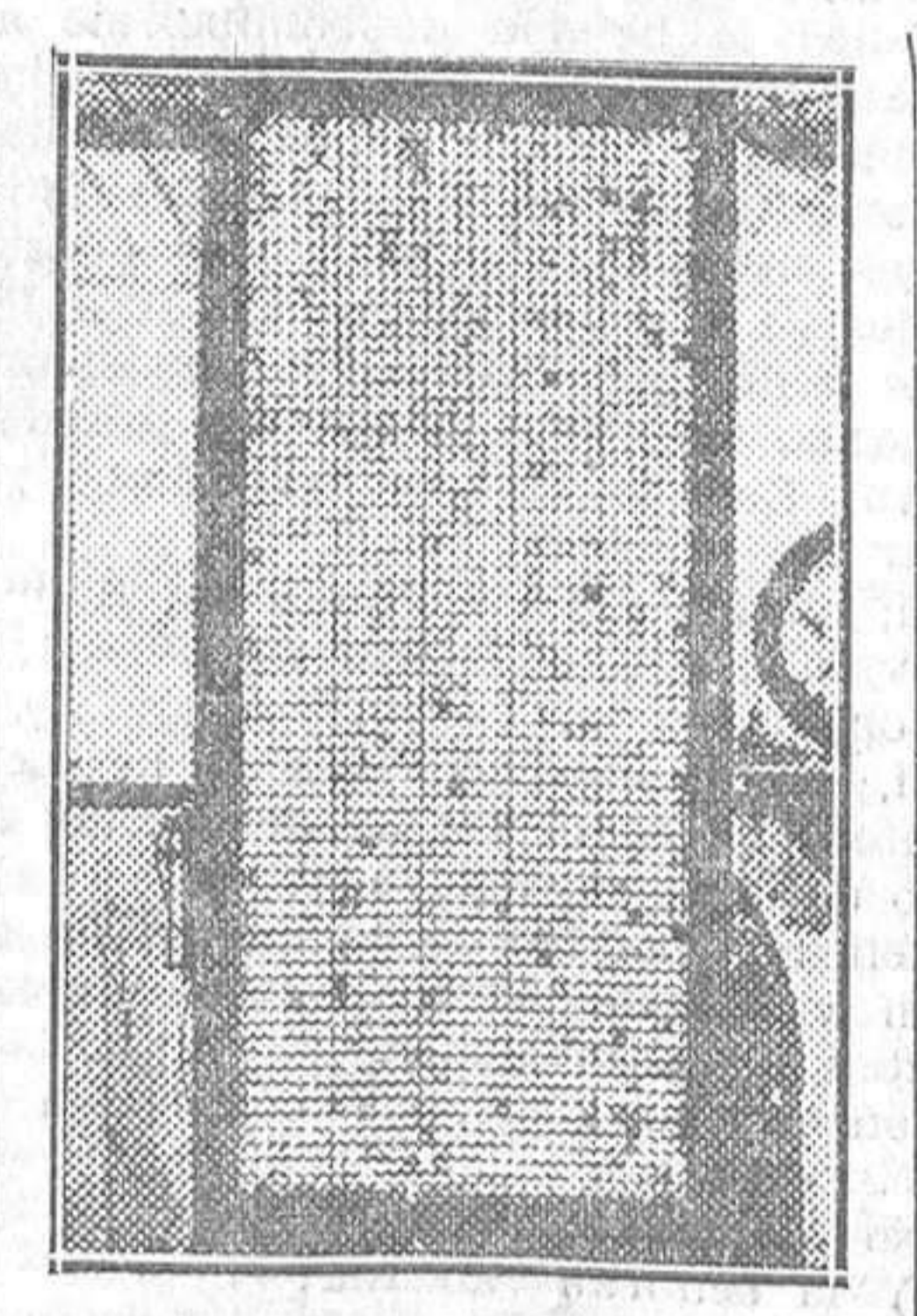
Pantalla de televisión para numerosos espectadores, usada en sus ensayos de televisión por la B. B. C. Se compone de más de dos mil pequeñas lámparas, en las que el grado de intensidad luminosa es variable, y se corresponde con la luz y sombra de la escena cuya transmisión a distancia se realiza.
