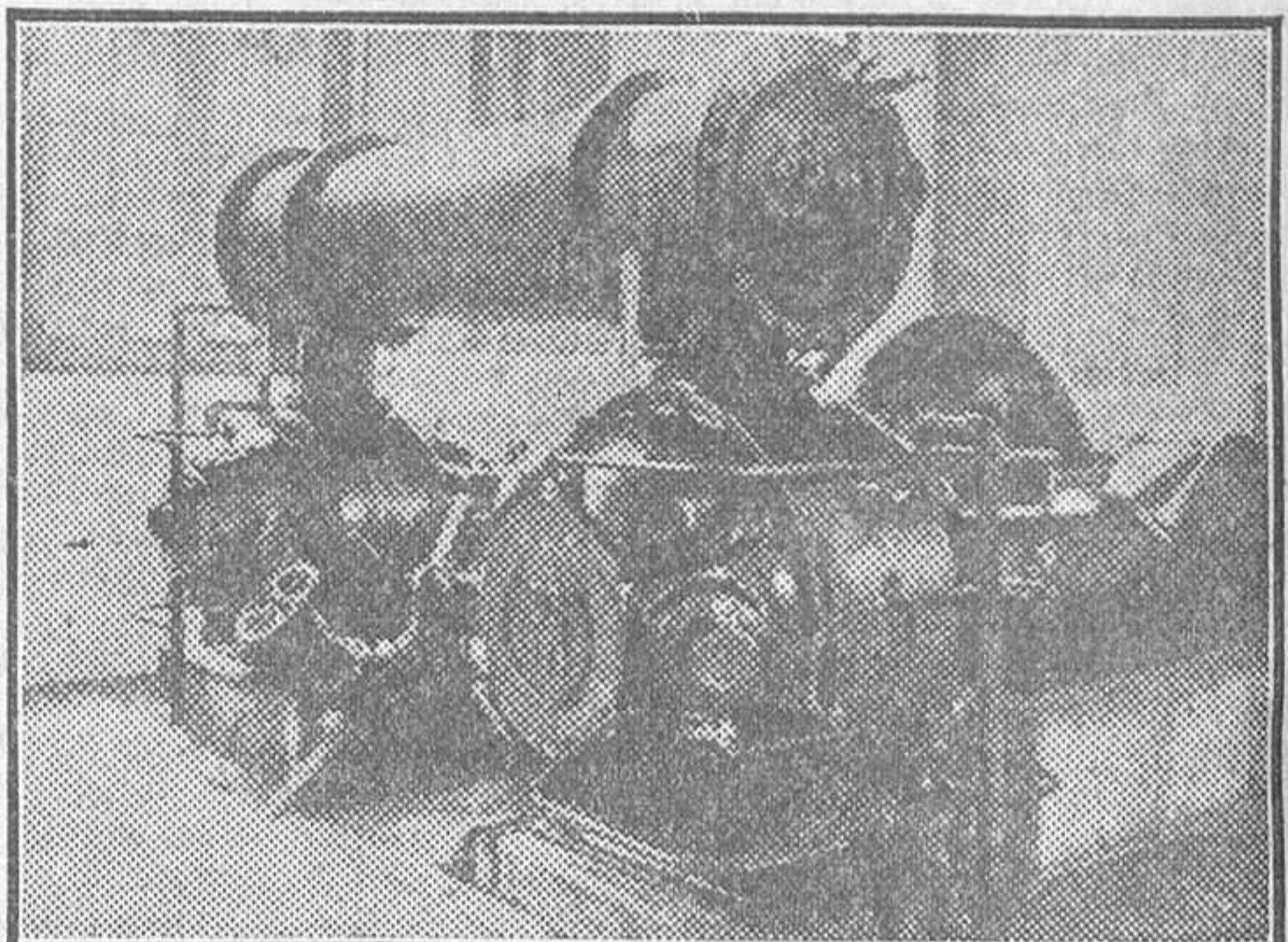
Compresor del grupo Santa Bárbara
