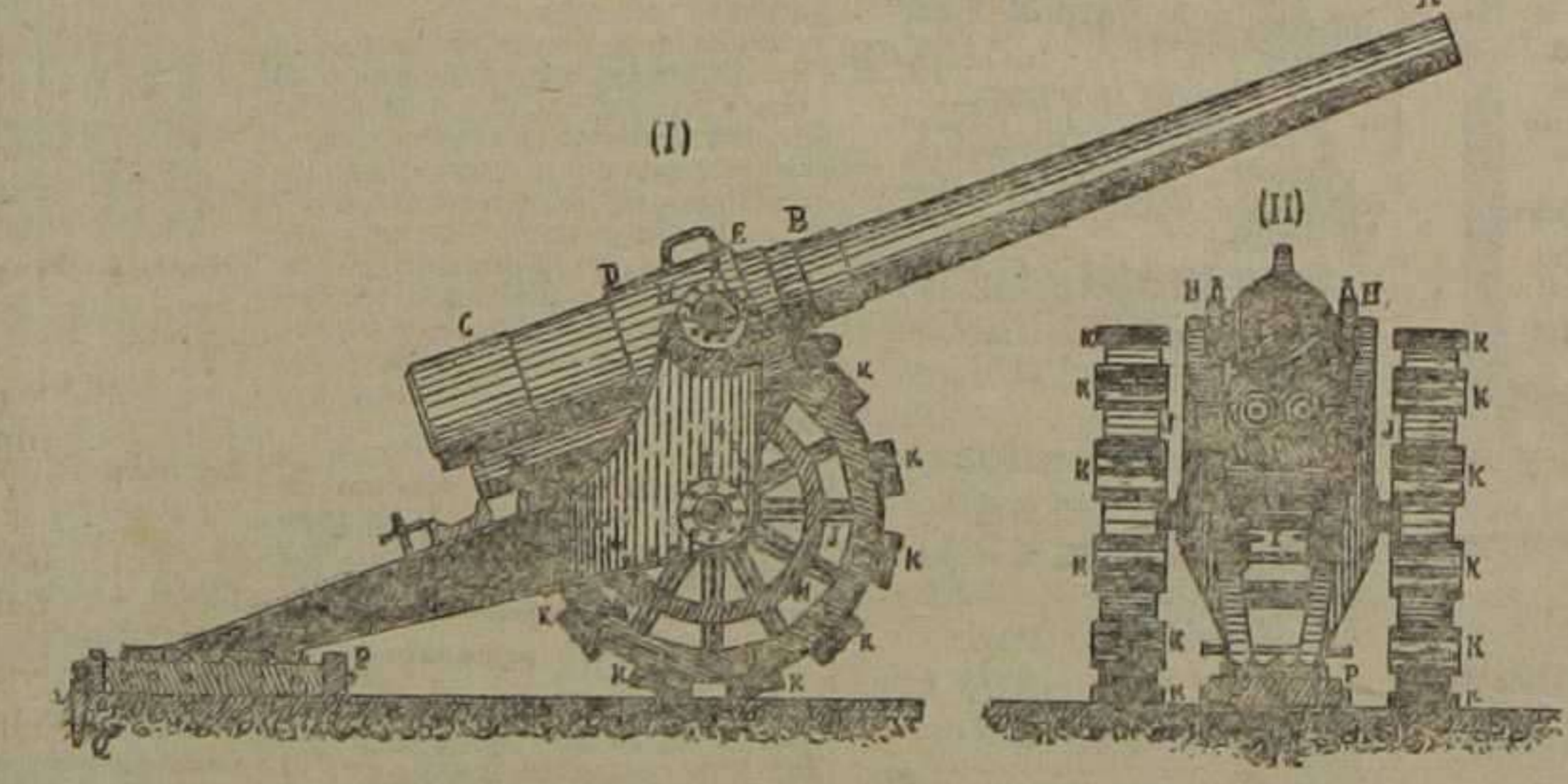
Figura 15.—Cañón de sitio de 15'5 centímetros, tipo largo de gran alcance, sistema «Schneider-Canet», sobre cureña de transporte. Modelo empleado por el ejército francés
